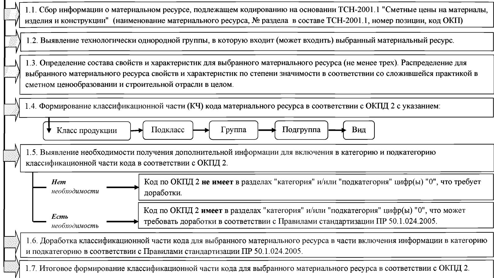
Рисунок 4.2. Последовательность формирования классификационной части кода материального ресурса
