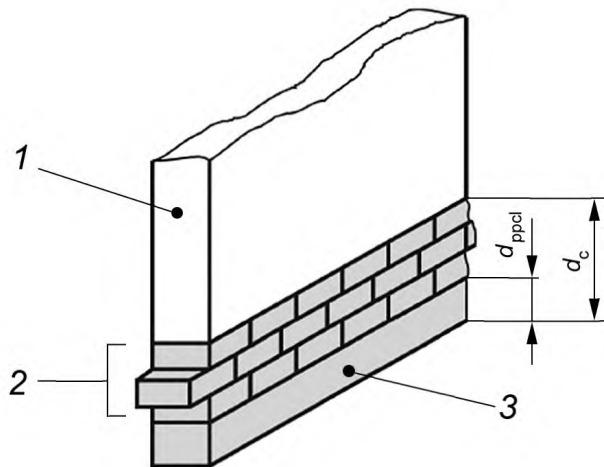
Рисунок 1 — Перемычка заводского изготовления (см. 3.1.19)
