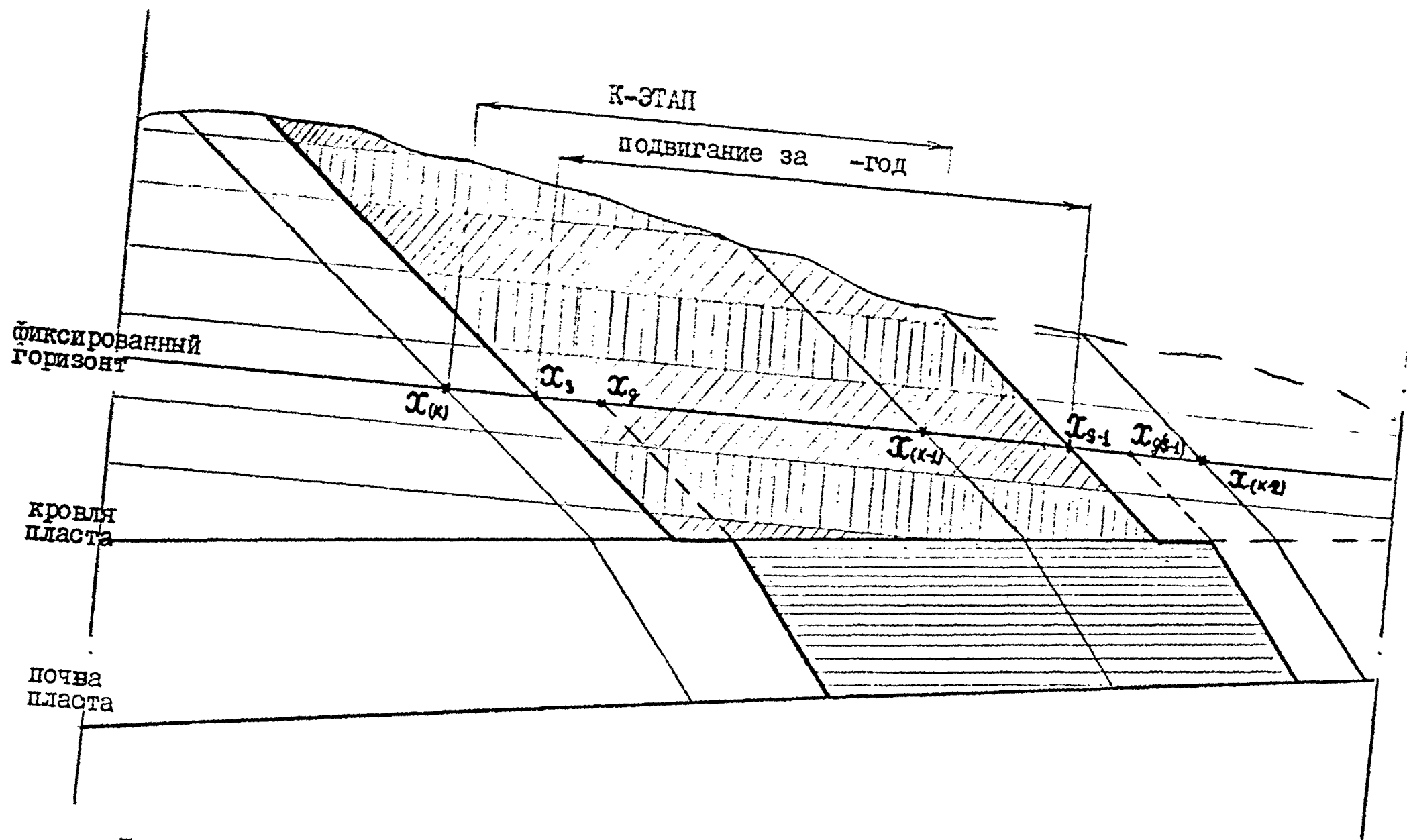
Рис. 27 Схема к расчету поуступных объемов угля и вскрышных пород.
