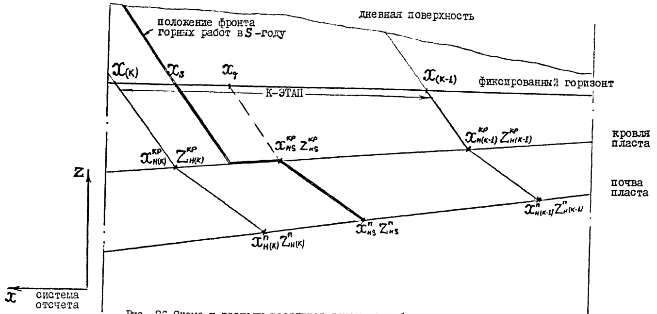
Рис. 36 Схема к расчету координат точек на добыче.
