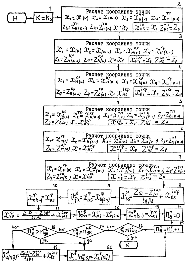
Рис. 33 Блок-схема алгоритма расчета координат характерных точек поперечных профилей на вскреше
