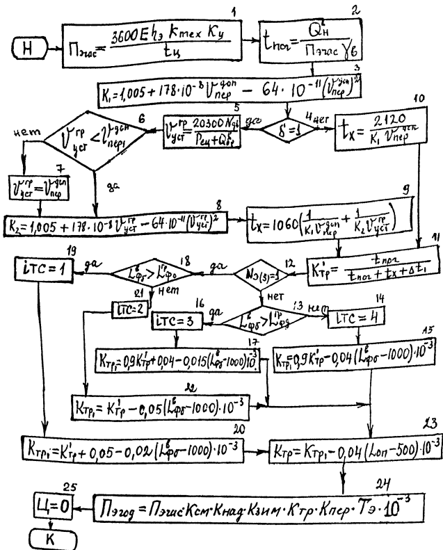
Рис. 22 Блок-схема алгоритма расчета производительности экскаватора на базисном этапе
