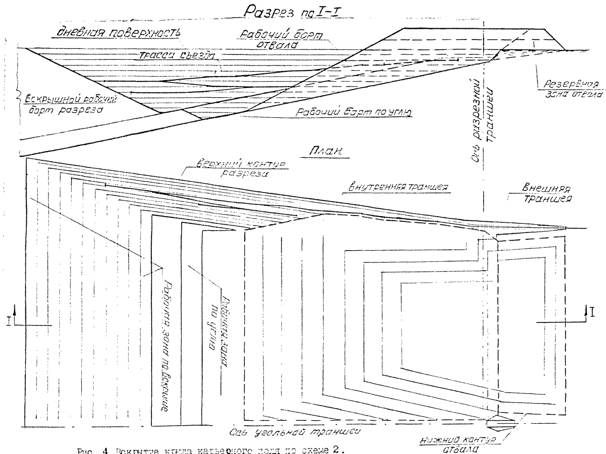
Рис. 4 Вскрытие края кафельного поля по схеме 2.
