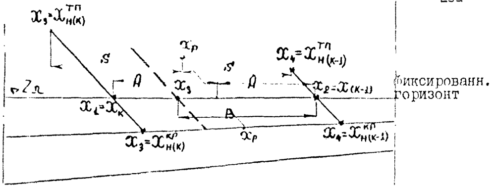
Рис. 7 Схема к расчету координат точек на профиле N.
