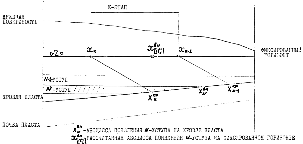
РИС. II СХЕМА К ПЕРЕСЧЕТУ АБСЦИССЫ НАЧАЛА УСТУПА НА КРОВЛЕ ПЛАСТА
