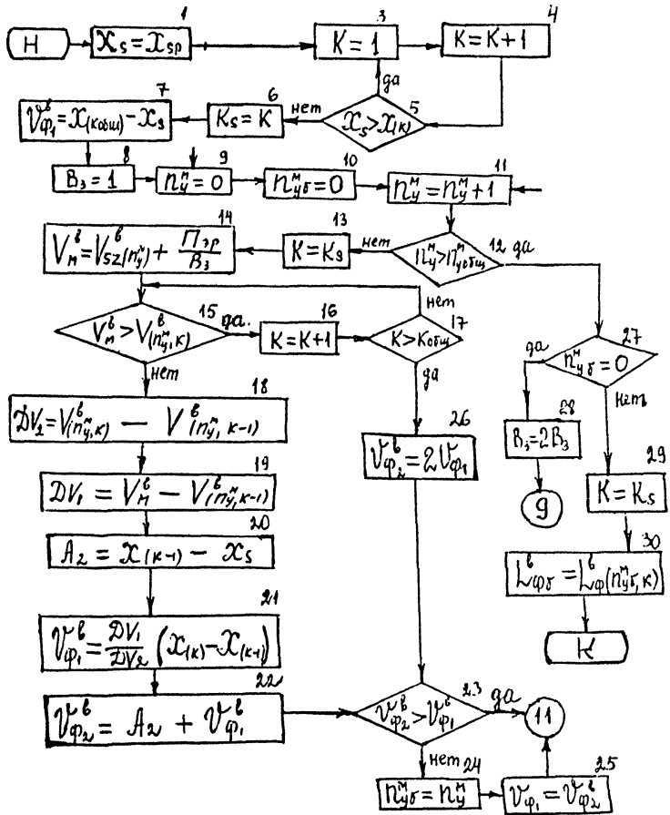
Рис. 21 Блок-схема алгоритма определения номера базисного уступа
