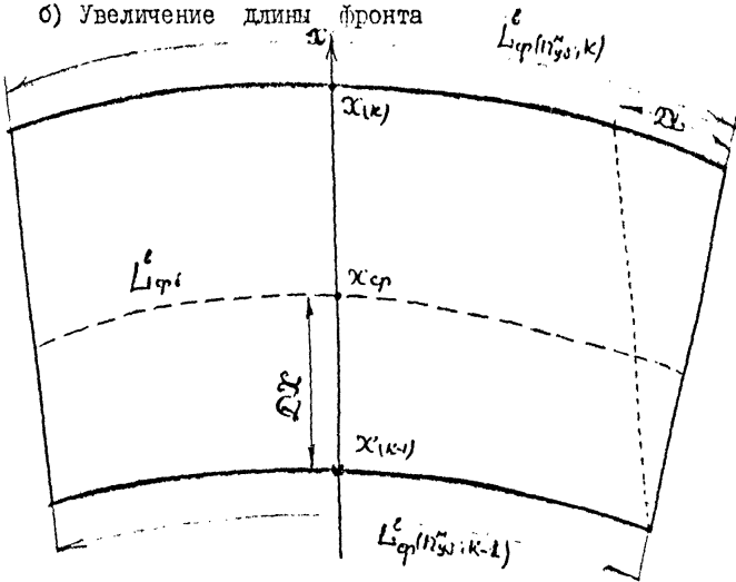
Рис. 25 Схема к расчету длины фронта базисного уступа на середину текущего года обработки.
