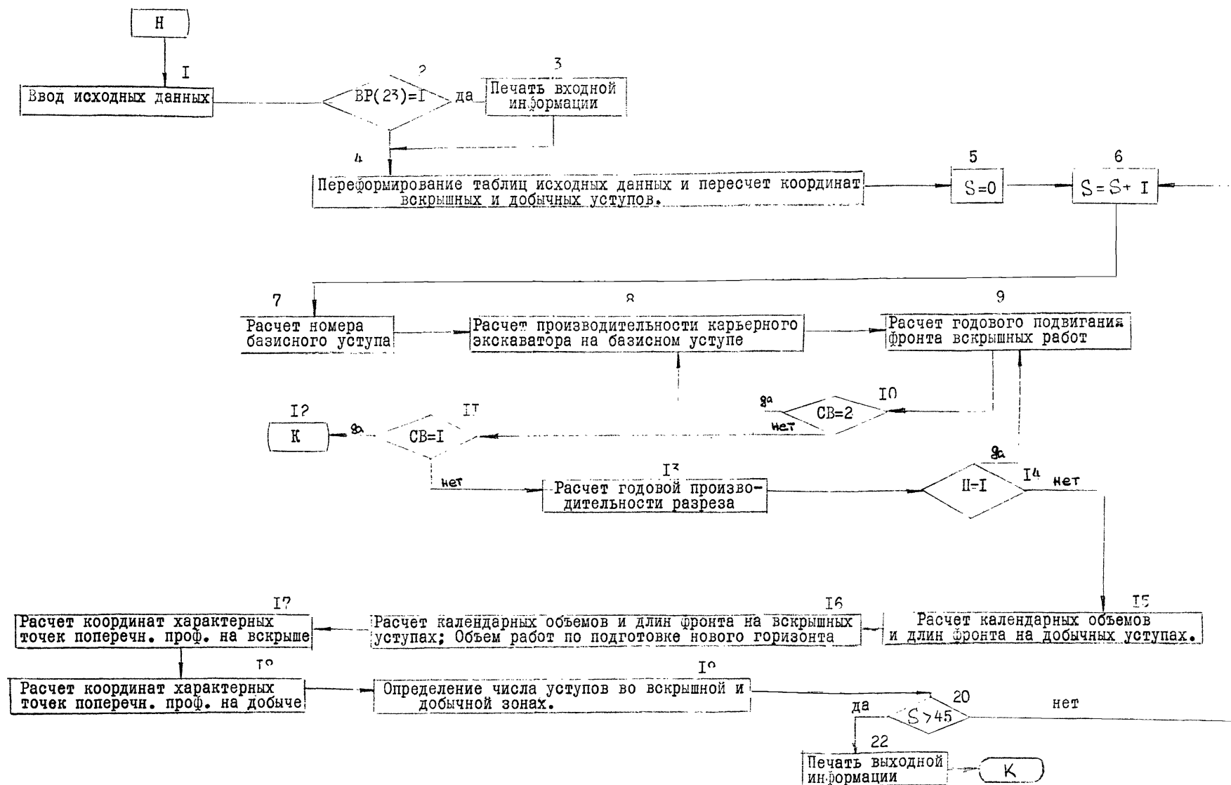
Рис. 5 Общая блок-схема алгоритма расчета интенсивности обработки карьерного поля.
