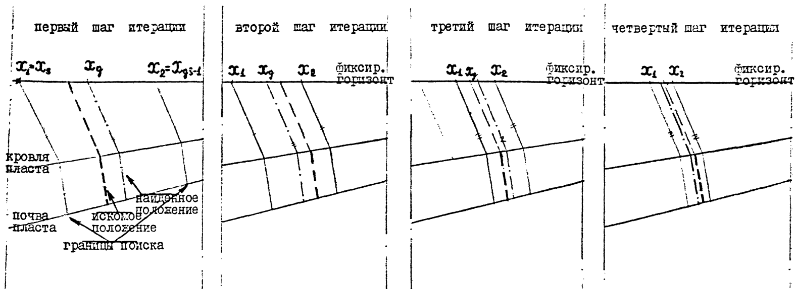
Рис. 29 Схема к расчету календарных объемов работ на добинных уступах.
