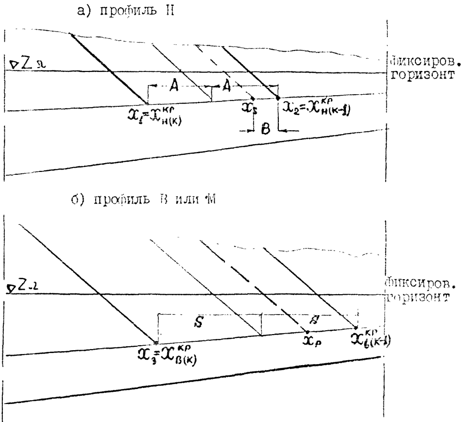
Рис. 8 Схема к расчету координат точек на поперечных B и M с использованием координат профиля N.
