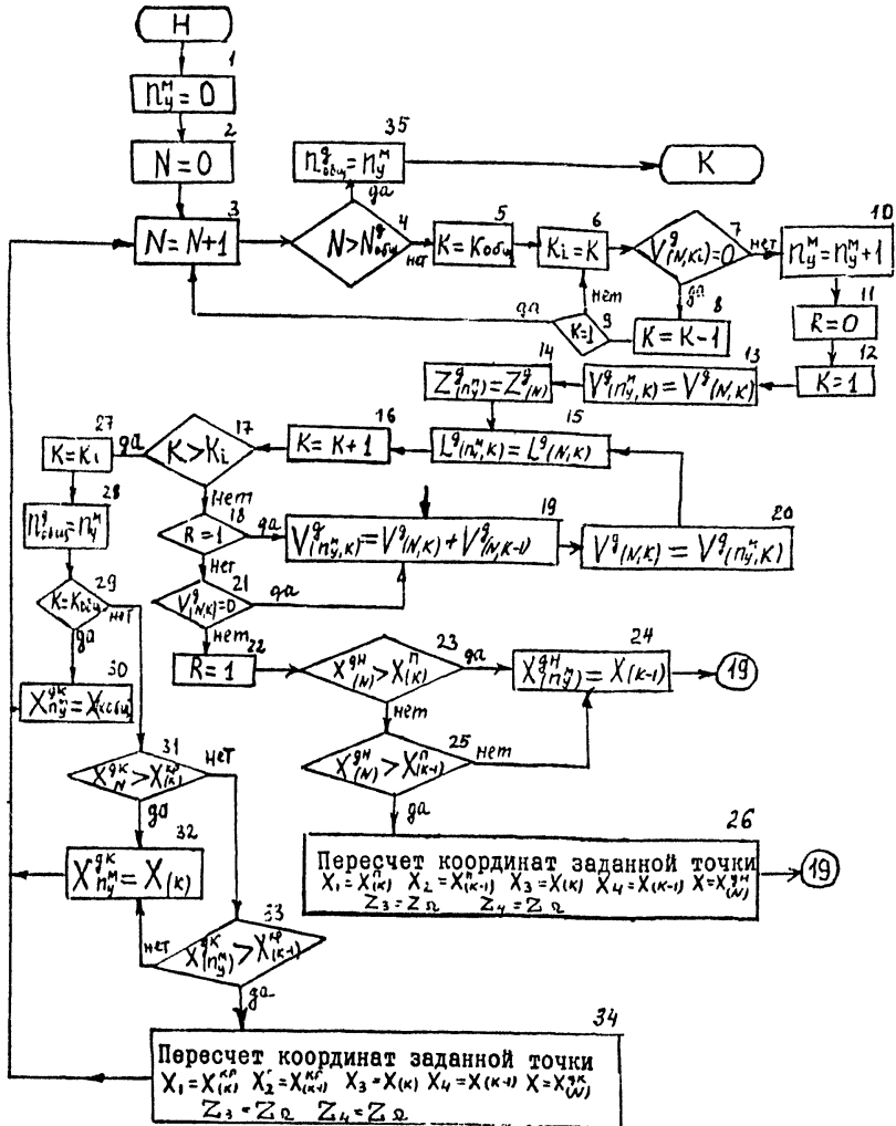
Рис. 15 Блок-схема алгоритма переформирования таблиц исходных данных и пересчета координат добычных уступов
