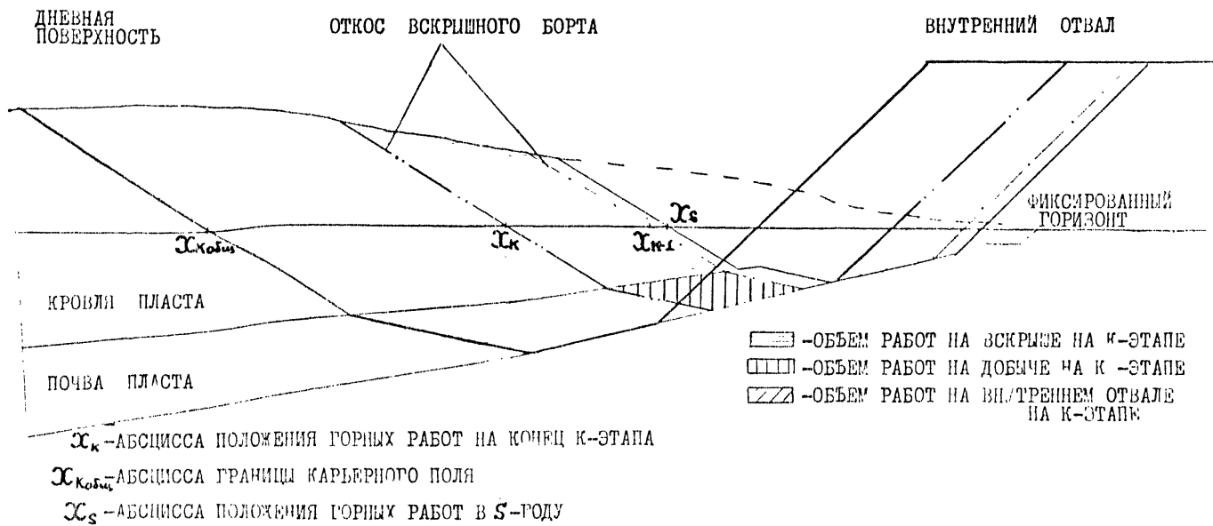
РИС.2 СХЕМА К ЭТАПНОЙ УВЯЗКЕ ПОЛОЖЕНИЯ ГОРНЫХ РАБОТ НА ВСКРЫШЕ, ДОБЫЧЕ И ОТВАЛЕ НА НАЗНАЧЕННОМ ПОПЕРЕЧНОМ ПРОФИЛЕ (ПРОФИЛЬ N).
