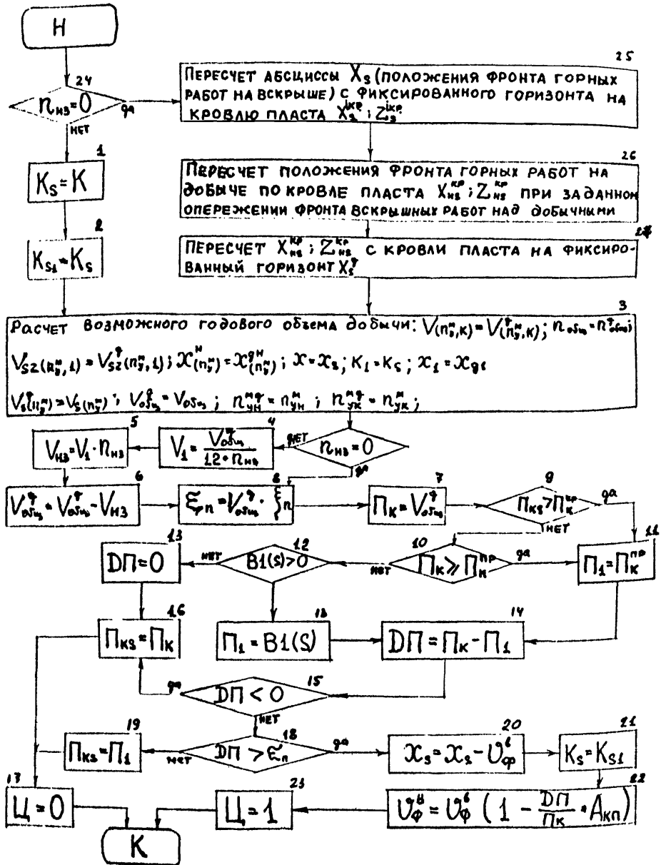
Рис. 28 Блок-схема алгоритма расчета производительности угольного разреза
