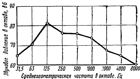
Черт. 2. Пример построения спектра внешнего шума легкового автомобиля.
