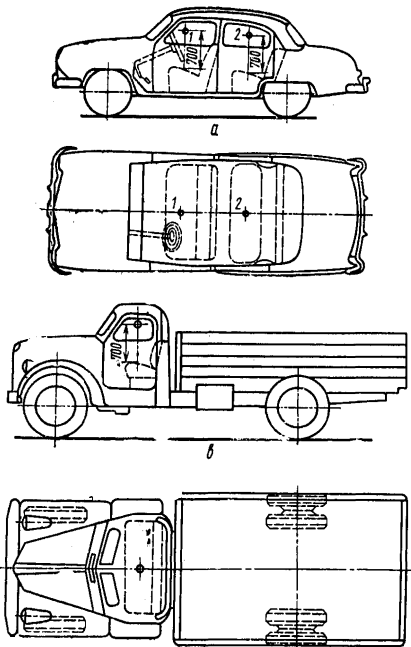
Черт. 3. Примеры расположения точек измерений шума: в легковом автомобиле (а), в автобусе (б) и в кабине грузового автомобиля (в).
