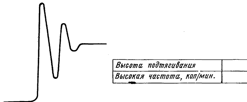
Черт. 13. Схематическая характеристика колебаний оси при подтягивании.
