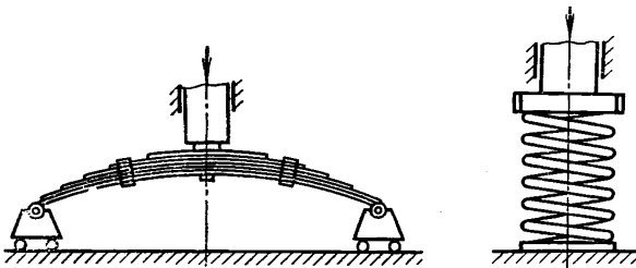
Черт. 16. Схемы тарировки рессор.
