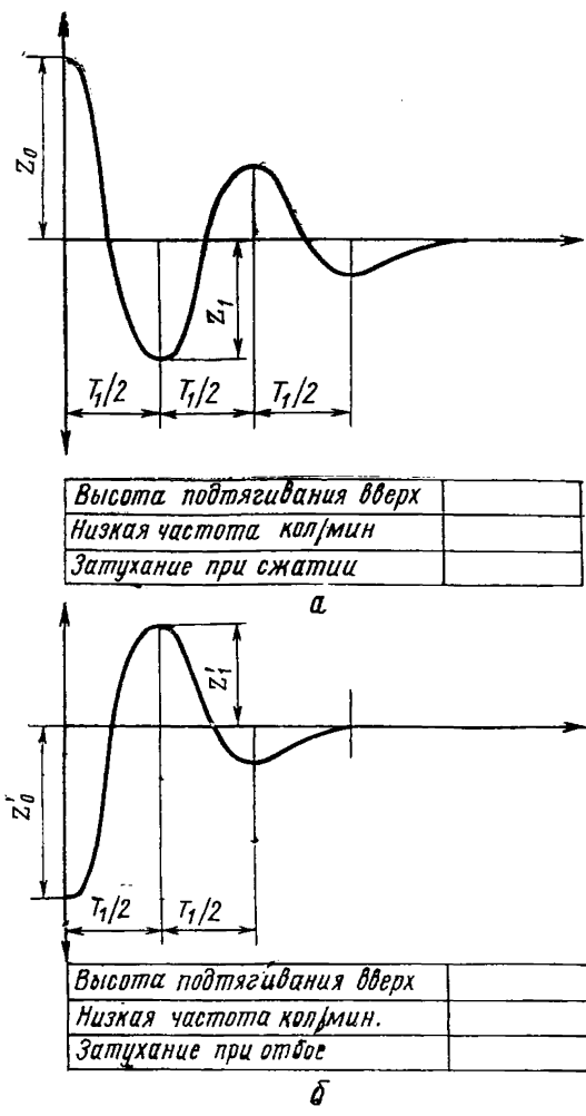
Черт. 12. Схематические характеристики колебаний кузова при подтягивании.
