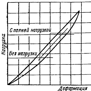
Черт. 19. Схематический график тарировки шин.
