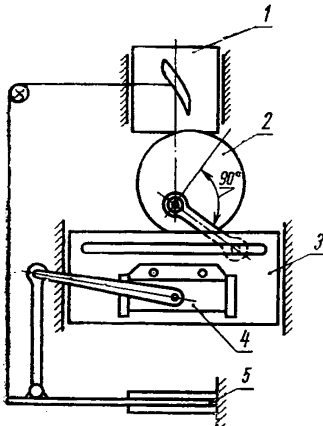
Черт. 20. Схема стенда для определения характеристик амортизаторов. 1 — панель для записи; 2 — эксцентрик; 3 — кулисный механизм; 4 — амортизатор; 5 — упругий элемент.
