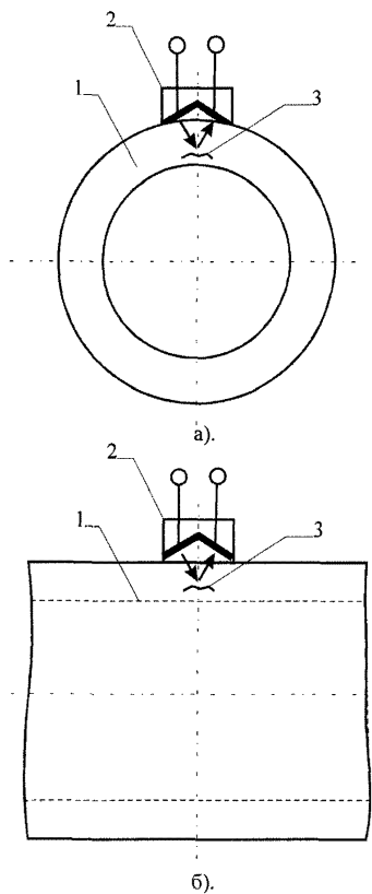
Рисунок А.1 - Схема УЗК прямым раздельно-совместным ПЭП в диаметральной плоскости (а) и осевой плоскости (б) трубы. 1 – труба; 2 – ПЭП; 3 – дефект (расслоение)
