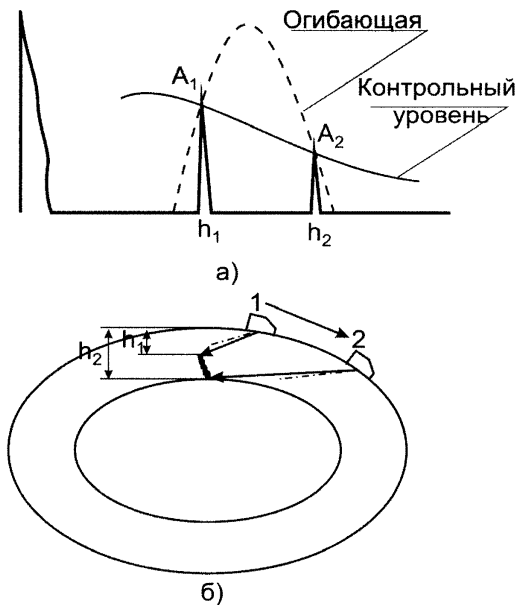
Рисунок 13 – Схема измерения условной высоты
