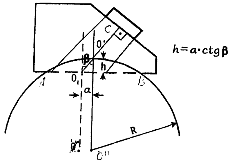
Рисунок В.2 - Разметка призмы преобразователя для сопряжения с изделием (второй способ)
