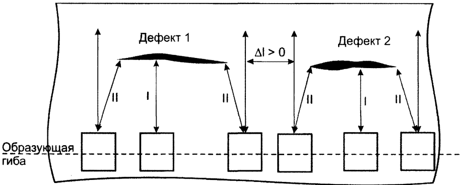
Рисунок 14 – Схема измерения условной протяженности
