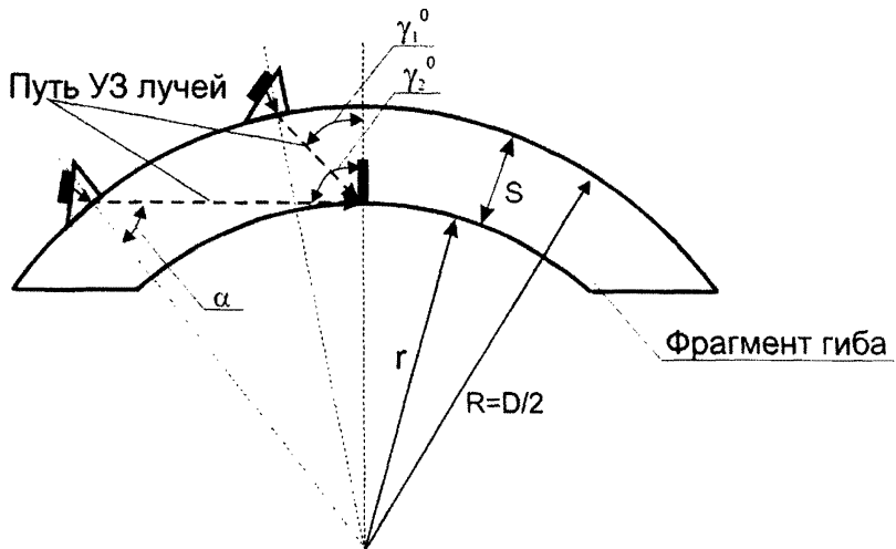
Рисунок 4 – Схема УЗК для \gamma_1 = 45^\circ и \gamma_2 = 90^\circ
