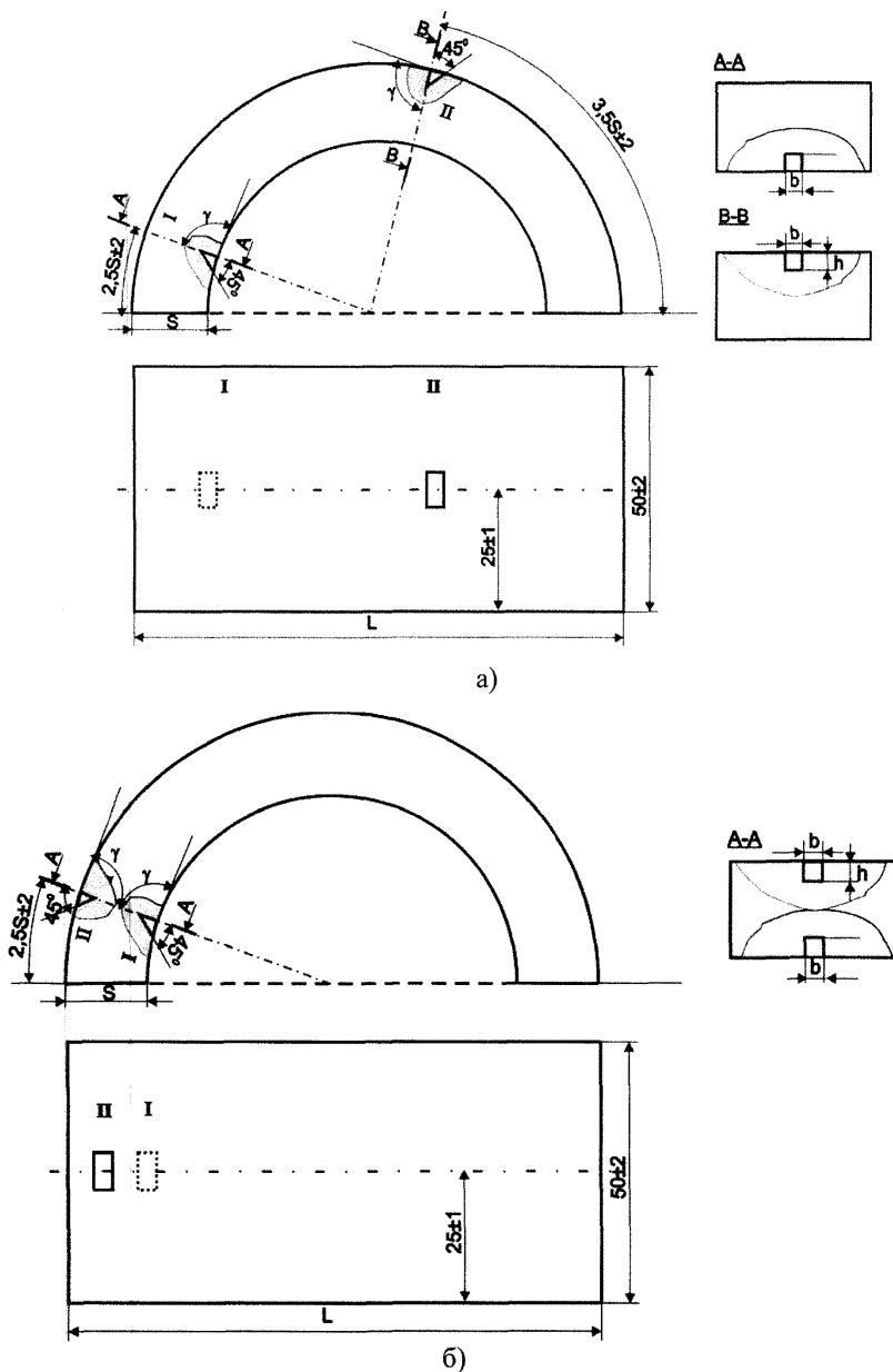
Рисунок 2 – Стандартный образец предприятия с зарубками для УЗК гибов труб толщиной: а - до 15 мм включительно, б – более 15 мм.
