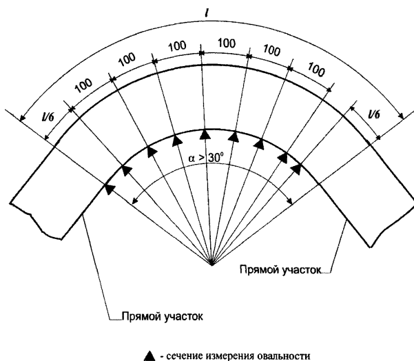
Рисунок 11 – Схема измерения овальностигиба
