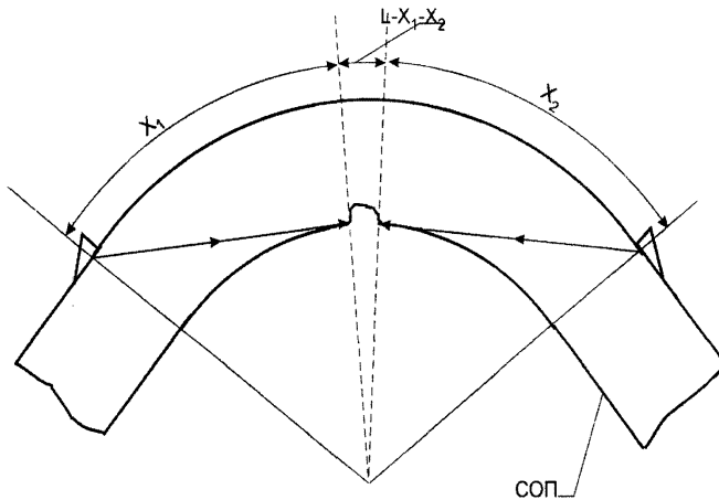
Рисунок 15 – Схема измерения условной ширины
