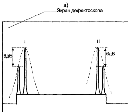
Рисунок 7 - Настройка скорости развертки а - схема хода лучей при настройке.
