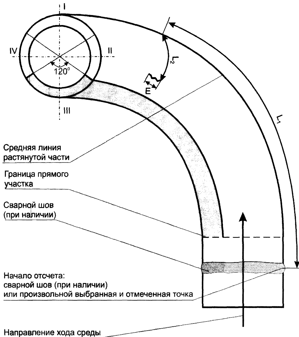
Рисунок 6 - Пример системы координат гiba
