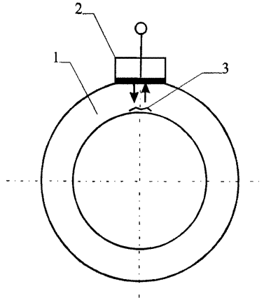
Рисунок А.2 - Схема УЗК прямым совмещенным ПЭП
