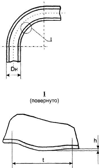
Рисунок 8 – Схема измерения волнистости на внутреннем обводегиба
