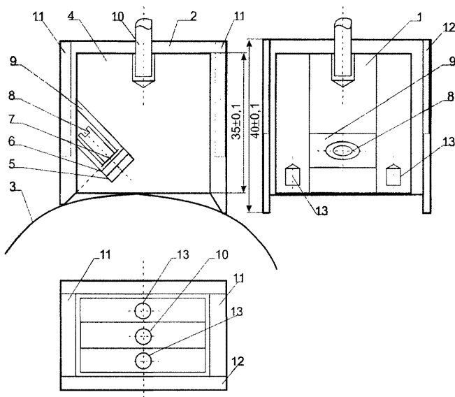
Рисунок Б.1 – Принципиальная схема обоймы
