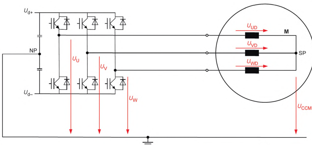
Рисунок А.1 — Схема инвертора и двигателя
