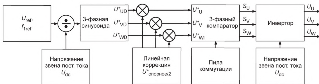
Рисунок А.2 — Структура системы формирования напряжения инвертора
