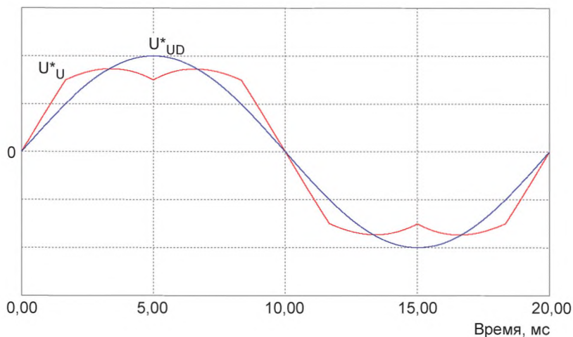
Рисунок А.4 — Заданное значение напряжения U_{UD}^* и модифицированное напряжение задания на входе компаратора
