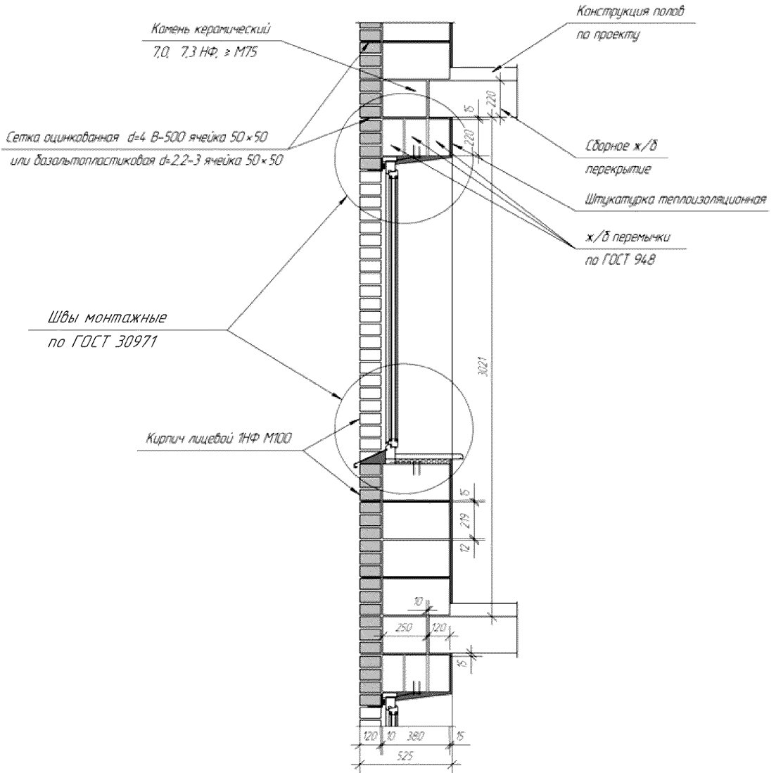
Рисунок А.7 – Тип 5, узел 2. Сборное железобетонное перекрытие
