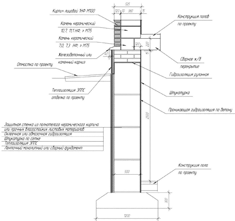
Рисунок А.8 – Тип 5, узел 3. Сборное железобетонное перекрытие
