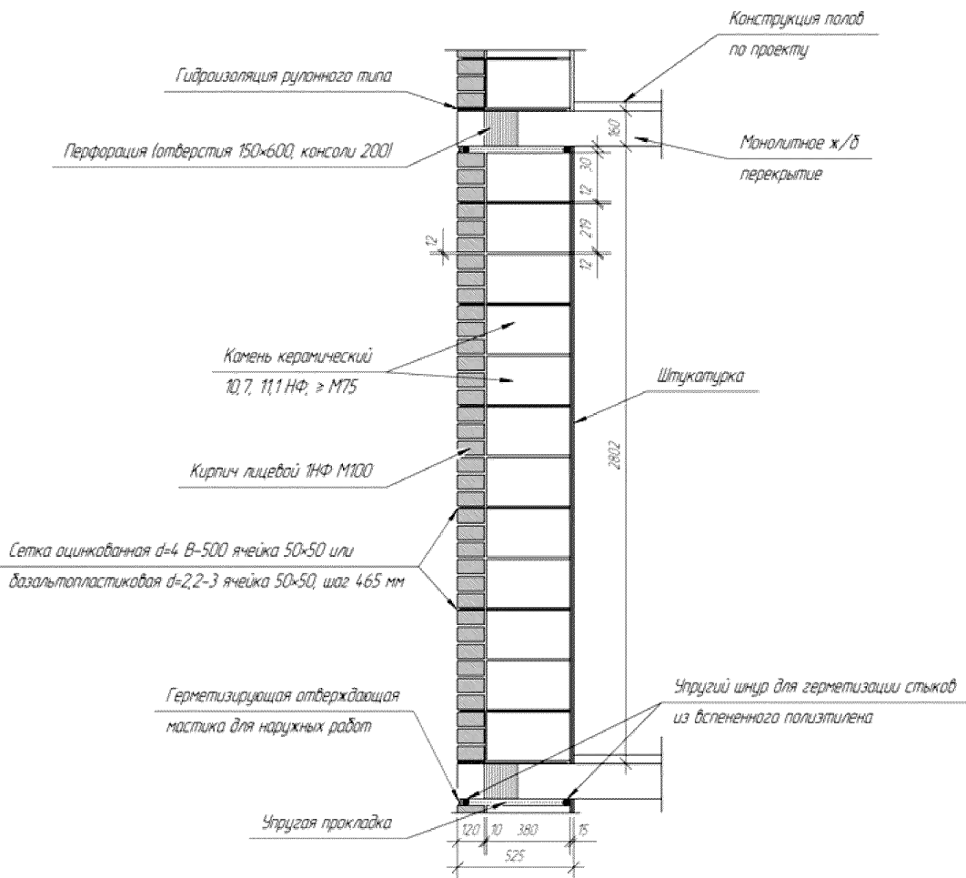
Рисунок Б.3 – Тип 5, узел 1. Монолитный железобетонный каркас
