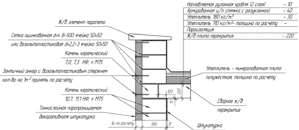
Рисунок А.13 – Тип 6, узел 4. Сборное железобетонное перекрытие
