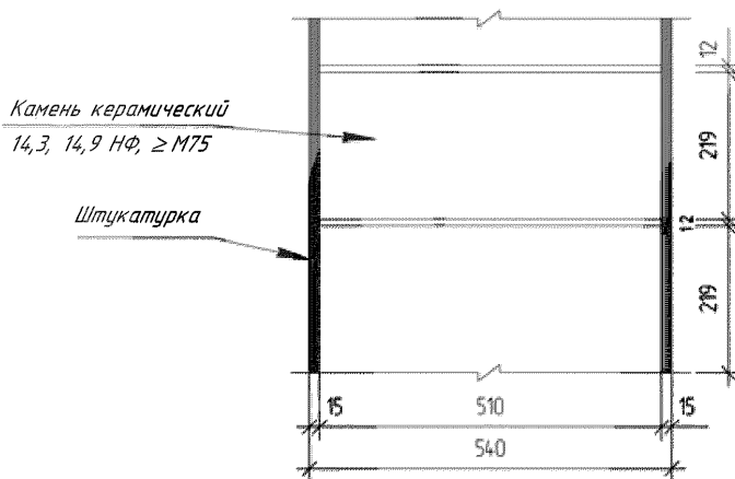
Рисунок В.1 – Однослойная стена из крупноформатных керамических камней толщиной 510 мм, оштукатуренная с двух сторон
