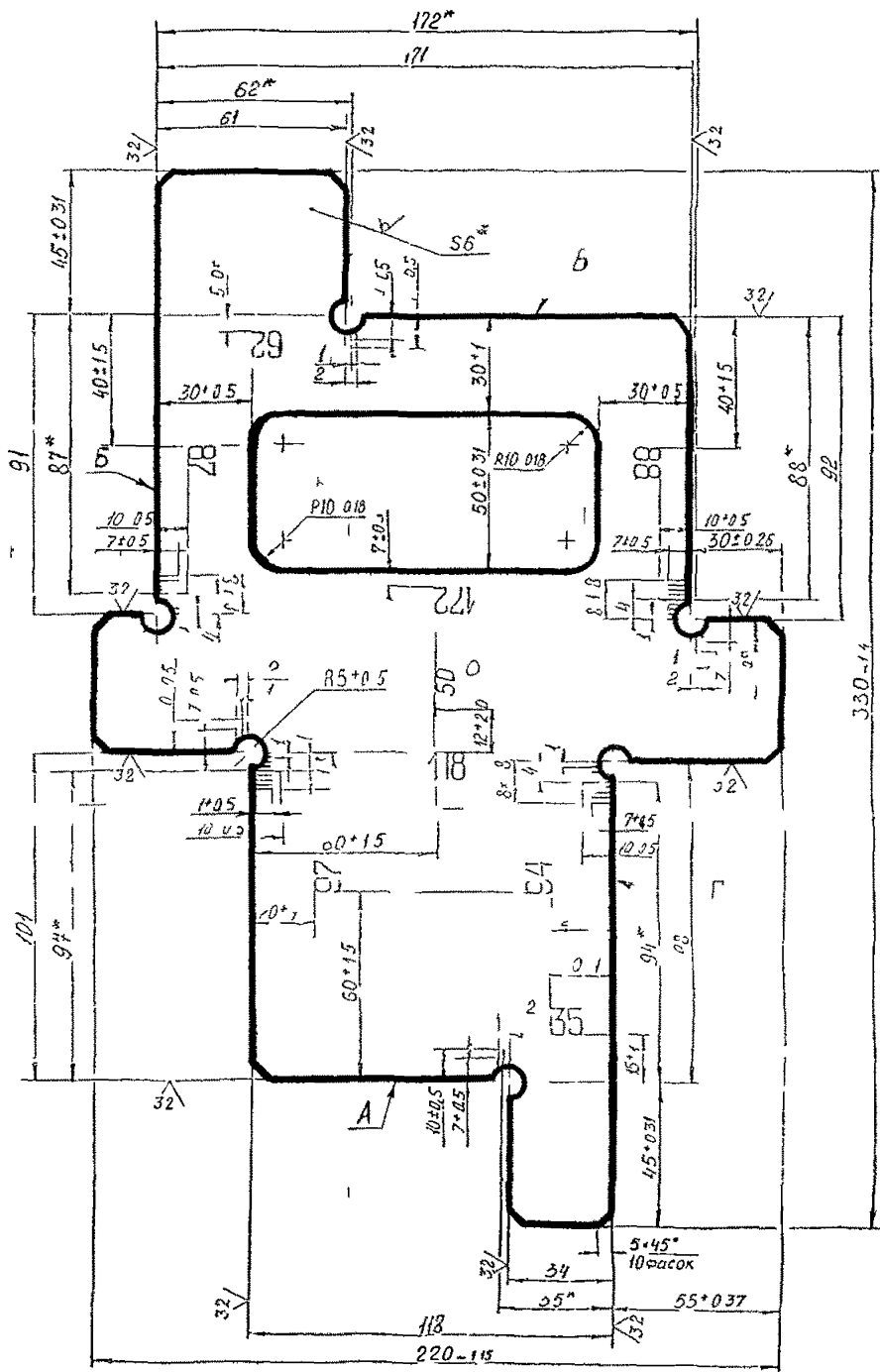
Рис. А в Модернизированный шаблон для контроля регулировок замедлителя Т-50.
