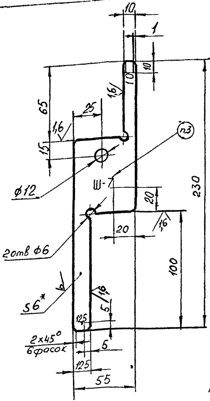
Рис. 66 Шаблон для контроля регуляторов замедлителя КВ-3.
