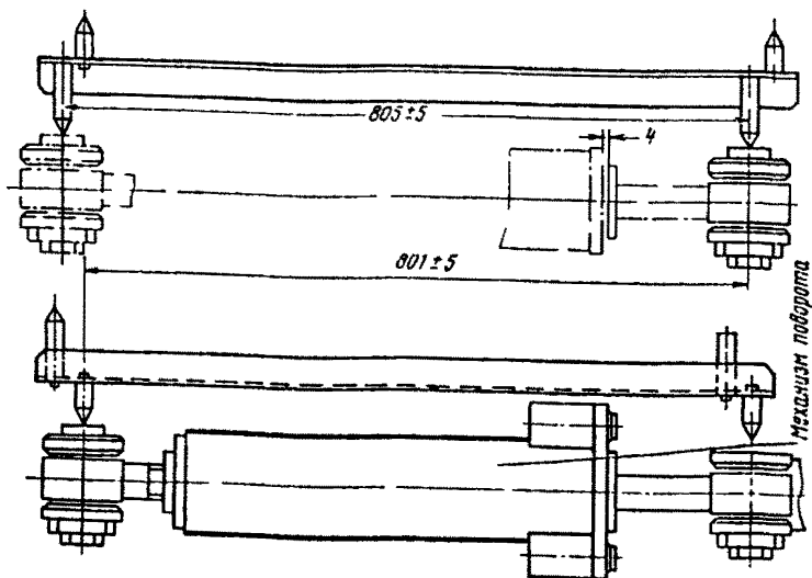
Рис. 611 Шаблон Ш-3 контроля межосевых расстояний механизма поворота замедлителя КВ
