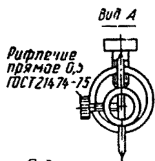
Рис. 612 Раздвижной шаблон для определения весового режима замедлителя КВ
