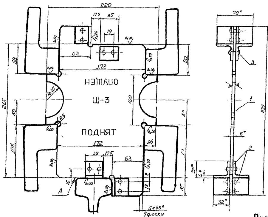
Рис. 640 Шаблон Ш-3 для контроля отторженного положения замедлителя КНН с механнизмом подъема
