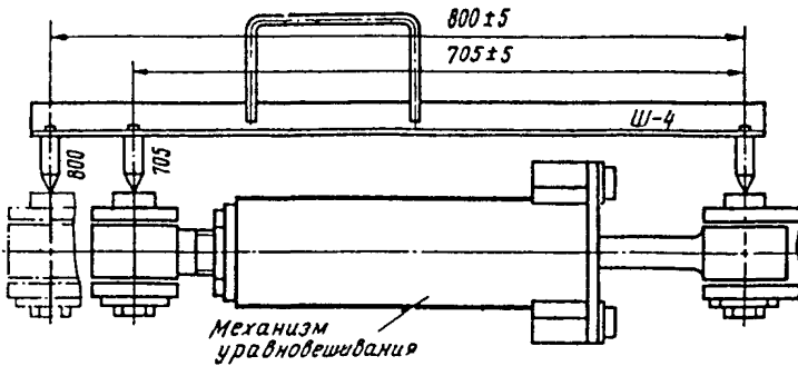
Рис. 514 Шаблон Ш-4 контроля межосевых расстояний механизма уравновешивания замедлителя КВ
