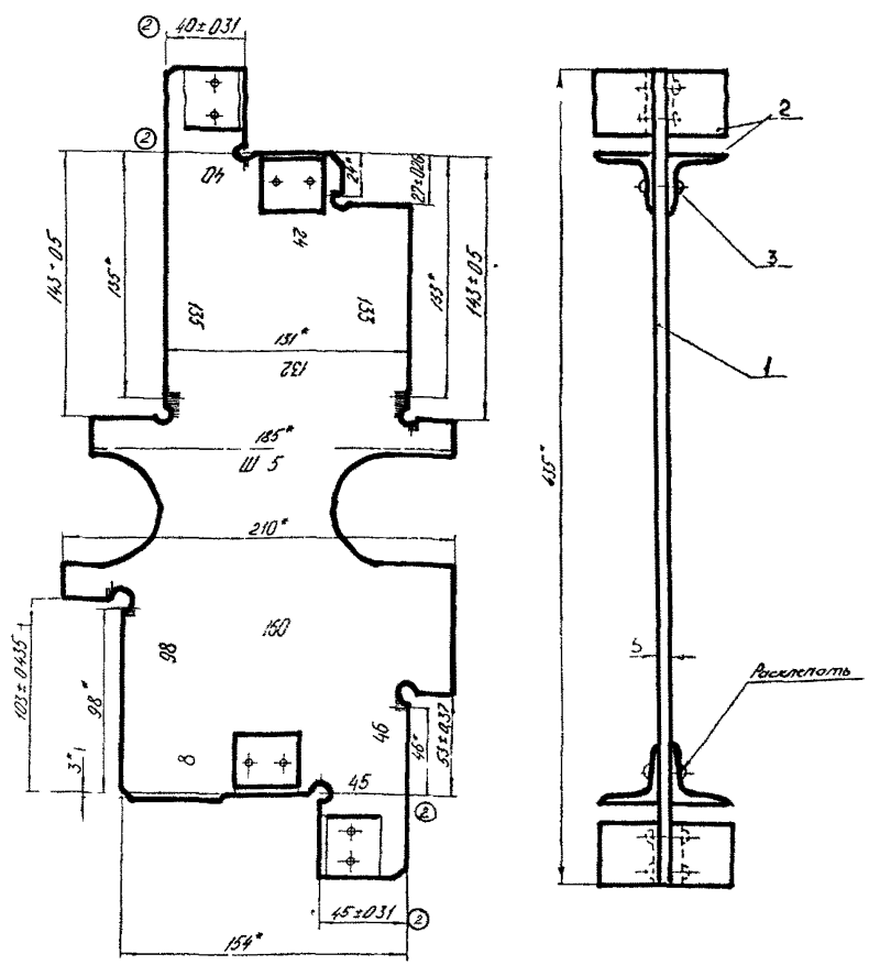
Рис. А3 Шаблон Ш-5 для контроля положений тормозных и подпорных шин замедлителя КВ.
