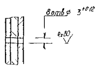
61 Рис. Б8 Шаблон для контроля подготов- ленного и тормозного положен- ний замедлителя ВЗПГ.
