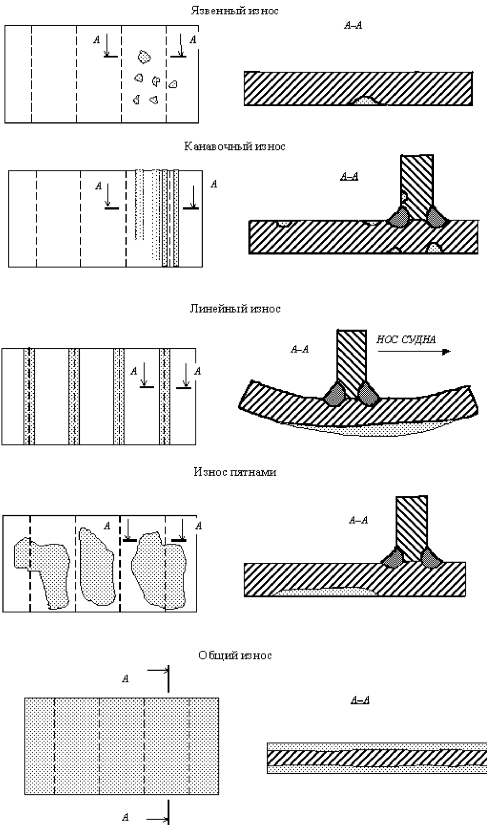
Рис. 1.2.1-2 Виды износов
