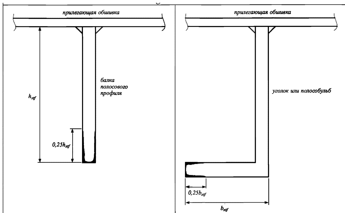
Рис. 1.2.1-5 Коррозия кромок
