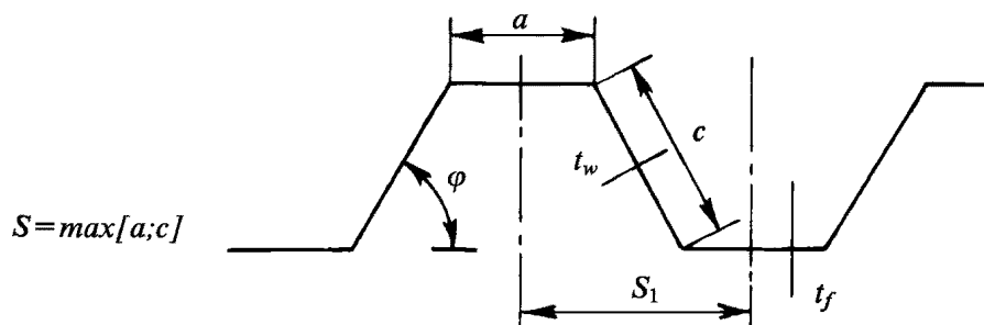
Рис. 5.9.2.3.1.1 Схема поперечной гофрированной переборки
