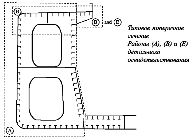
Типовое поперечное сечение Районы (А), (В) и (Е) детального освидетельствования
