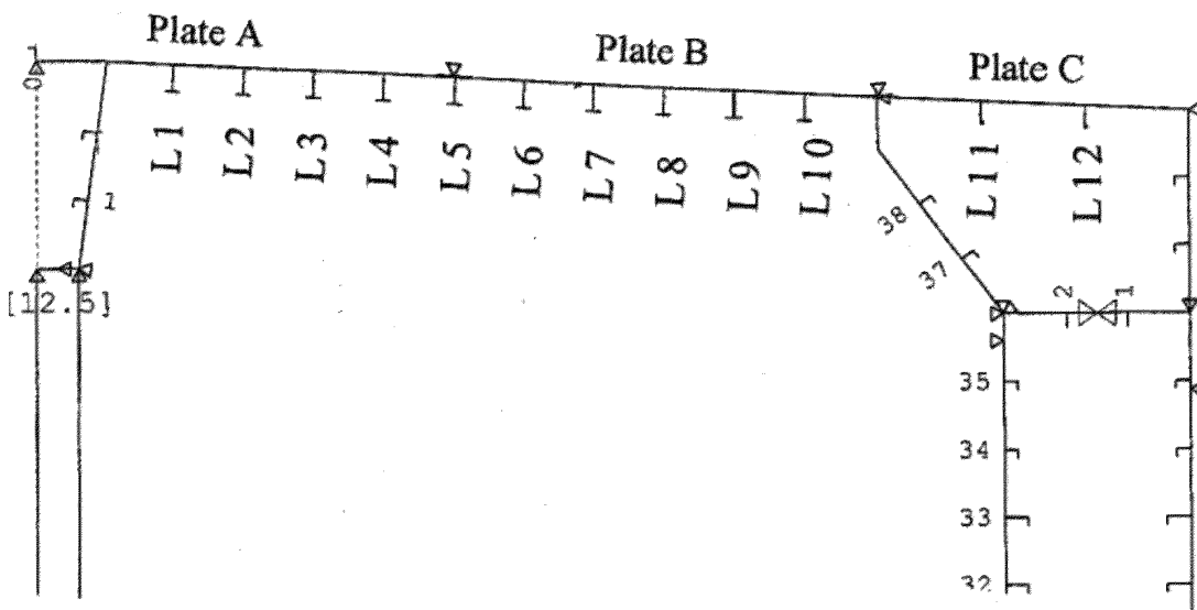
Рис. 1 Схема сечения половины ширины палубы судна
