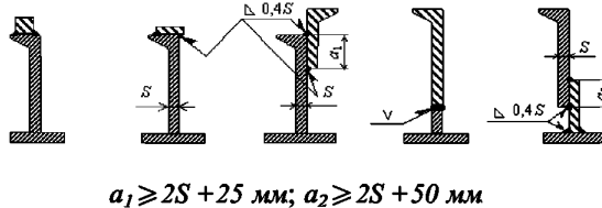
Рис. 5.2.4.1-1 Подкрепления балок набора:
