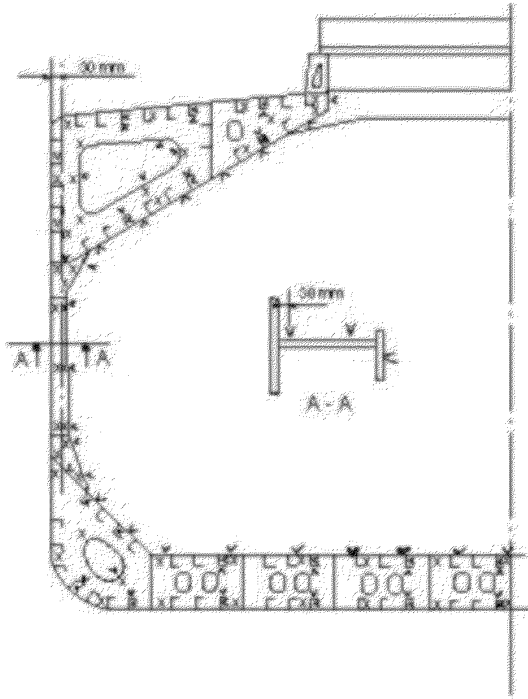
Рис. 5.3.6.1 Схема замеров поперечного набора на навалочных судах
