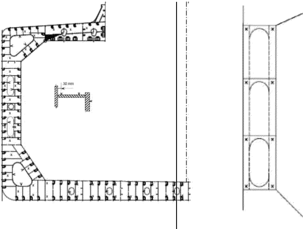
Рис. 5.3.6.1 Схема замеров поперечного набора на навалочных судах
