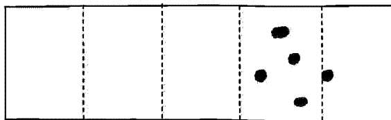
Рис. 5.4.3 Язвенная коррозия с интенсивностью 1 % и менее (единичные язвины в пределах ячейки листа)
