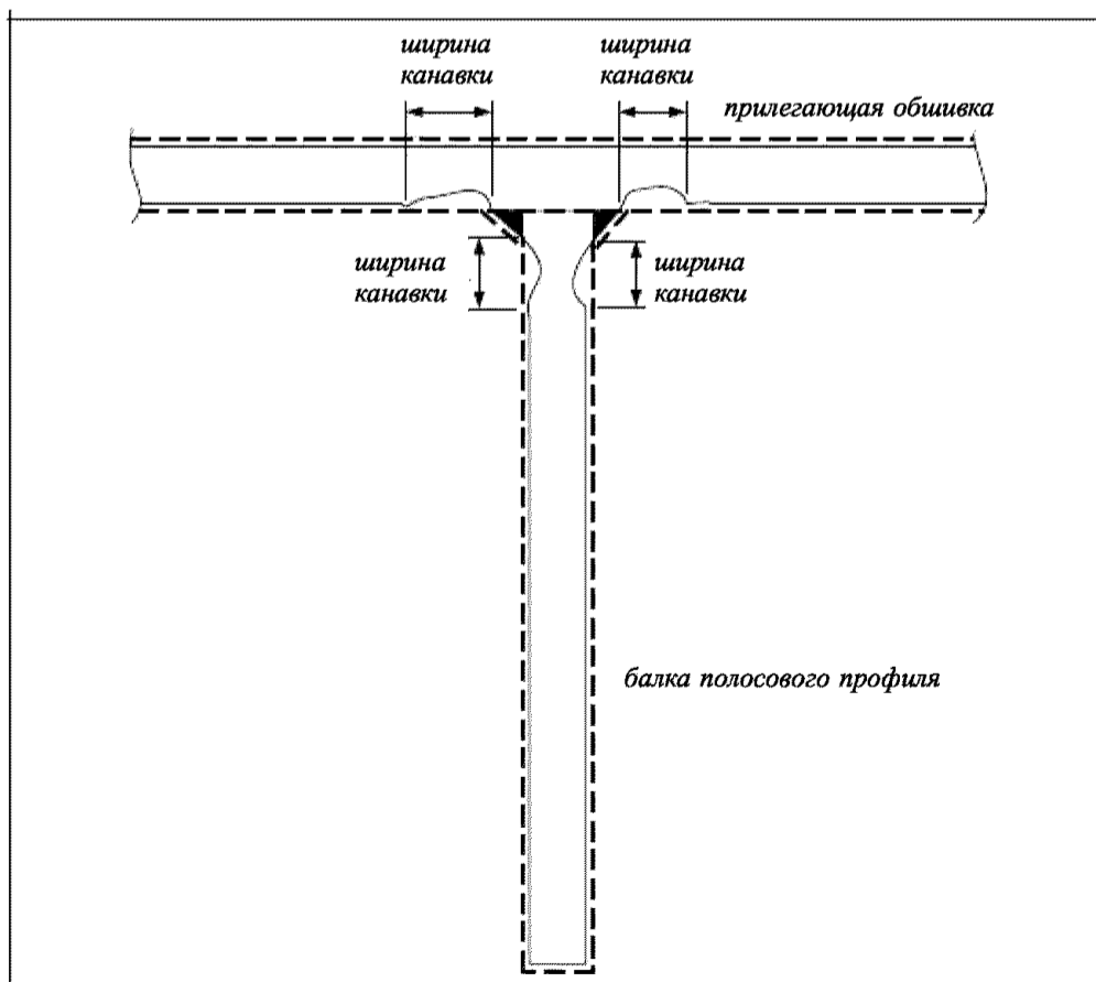
Рис. 1.2.1-4 Канавочный износ
