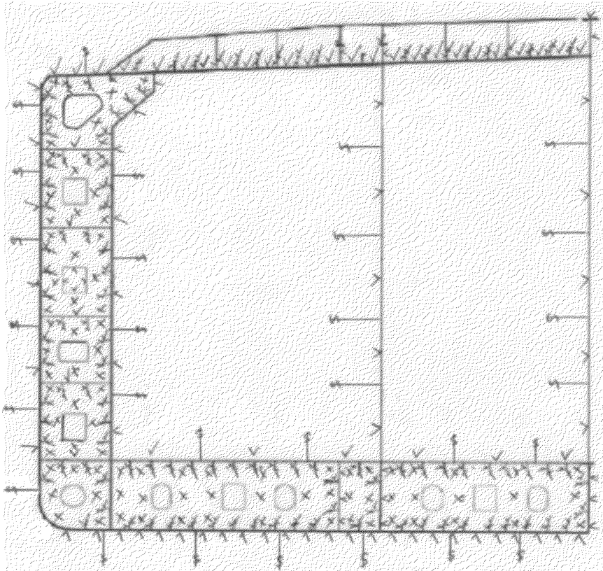
Рис. 5.2.6 Схема замеров в поперечном сечении танкера-химовоза
