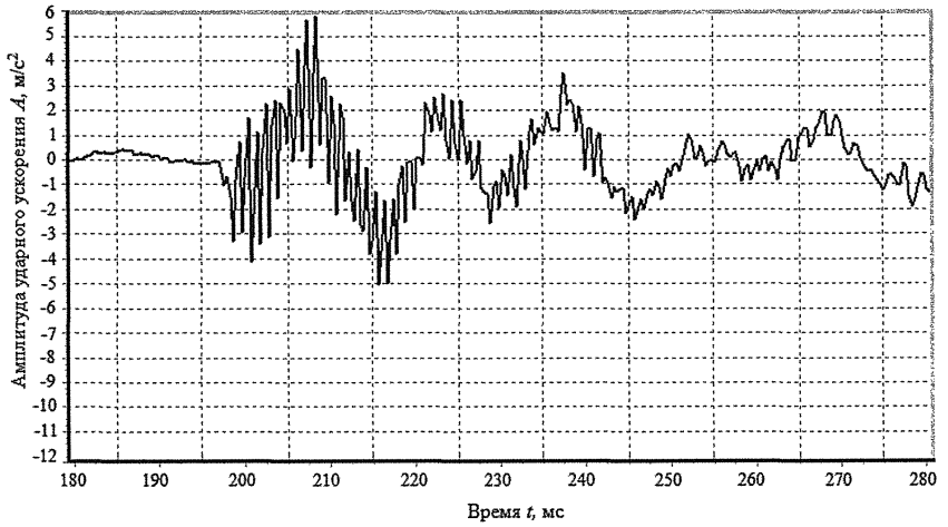
Рисунок Д.5– Ось OZ. Точка 4. Акселерограмма ударного воздействия
