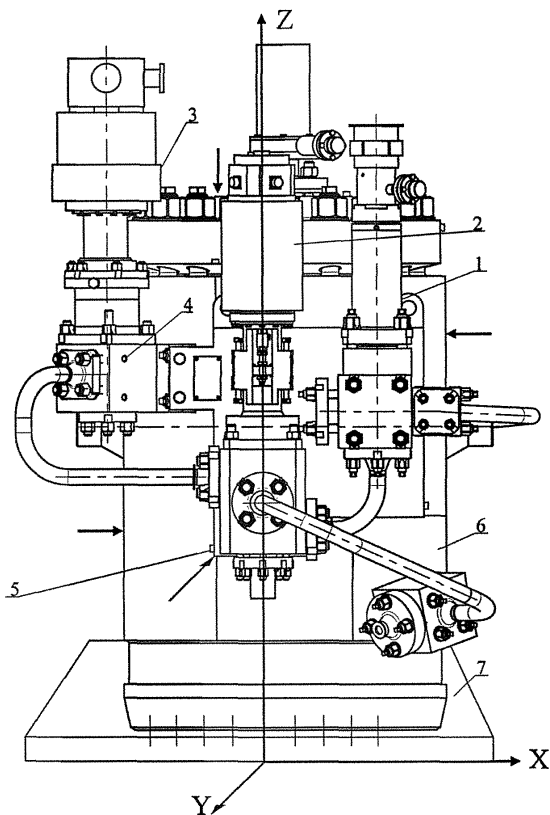
1, 2, 3, 4 – места (точки) установки вибропреобразователей; 6 – клапан; 7 – монтажная плита → – направление нанесения ударов
