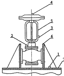
а) установочное положение арматуры приводом вверх, крепление арматуры к платформе с помощью угловых опор
