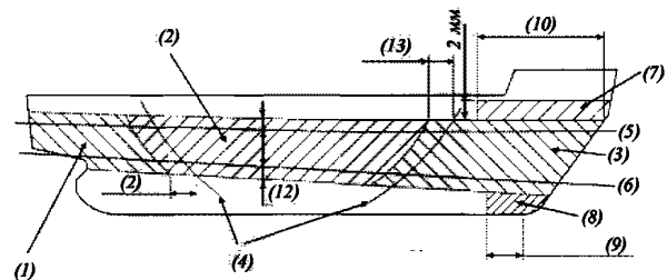
Рис. 10.5.1.1 Районы ледовых усилений корпуса судна: 1 — кормовой район; 2 — средний район; 3 — носовой район; 4 — линия плоского борта; 5 — ВЛВЛ; 6 — НЛВЛ; 7 — верхний носовой ледовый пояс; 8 — нижняя часть форштевня; 9 — 5 расстояний между балками основного набора; 10 — 0,2L ; 11 — см. 10.5.1; 12 — см. 10.5.3.1; 13 — см. 10.5.1
