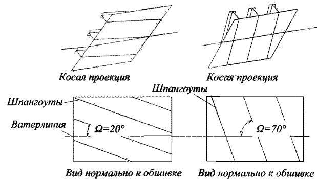
Рис. 1.2.4.2 Угол наклона Ω набора наружной обшивки
