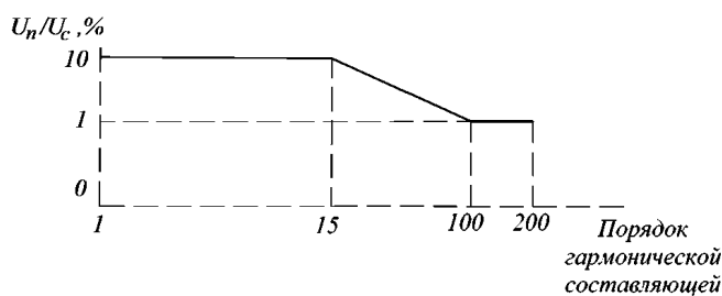
Рис. 2.2.1.2.2 График высших гармонических составляющих судовой сети
