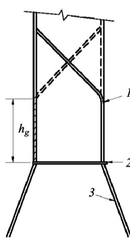
Рис. 4.2-3 Симметричные гасетные/шеддерные листы: 1 — гасетный/шеддерный лист; 2 — горизонтальный/наклонный лист опоры (полки) нижней опоры для переборки; 3 — вертикальная/наклонная стенка нижней опоры для переборки.
