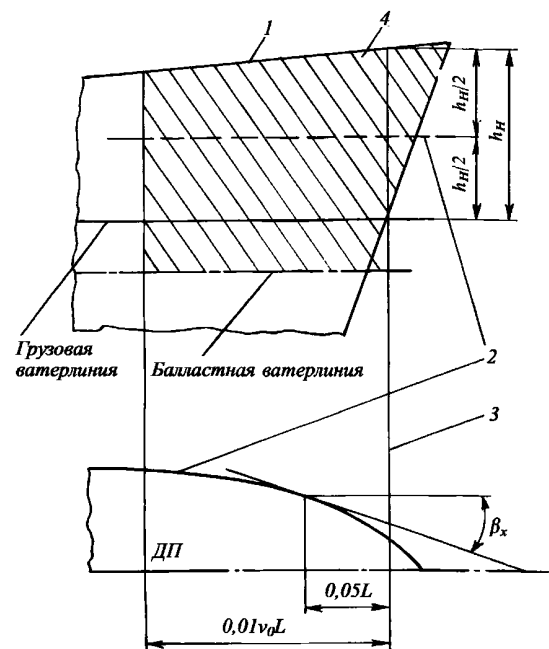
Рис. 2.8.1.2-2 Схема определения угла \beta_x и области действия ударного давления волн (затрихована): 1 — верхняя открытая палуба; 2 — ватерлиния для определения угла \beta_x ; 3 — носовой перпендикуляр; 4 — область ударных давлений;
