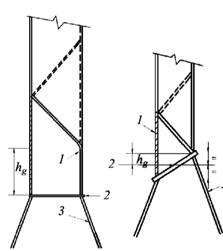
Рис. 4.2-4 Несимметричные гасетные/шеддерные листы: 1 — гасетный/шеддерный лист; 2 — горизонтальный/наклонный лист опоры (полки) нижней опоры для переборки; 3 — вертикальная/наклонная стенка нижней опоры для переборки.
