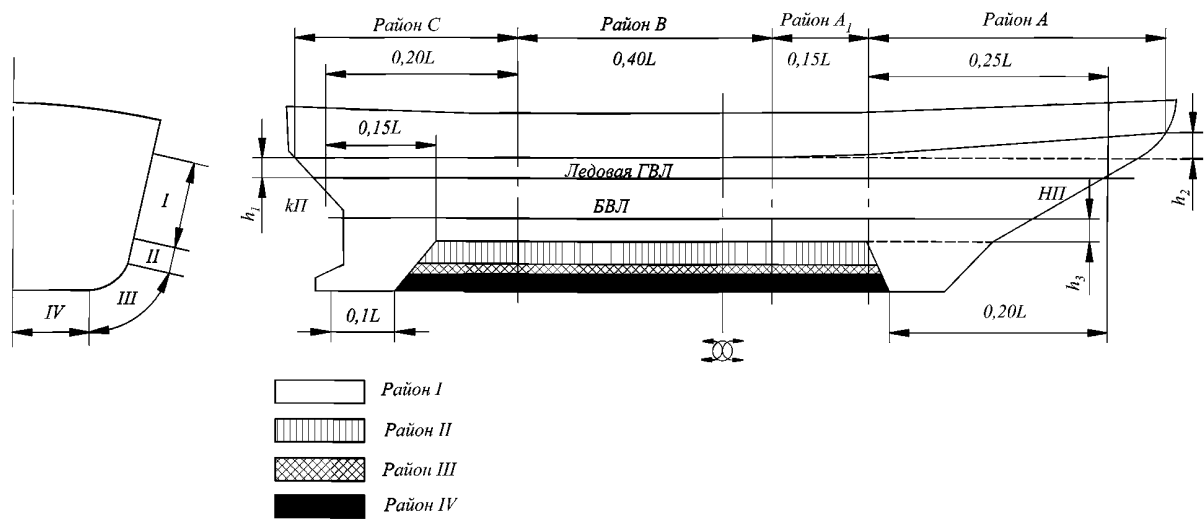
Рис. 3.10.1.3.3 Районы ледовых усилений ледоколов
