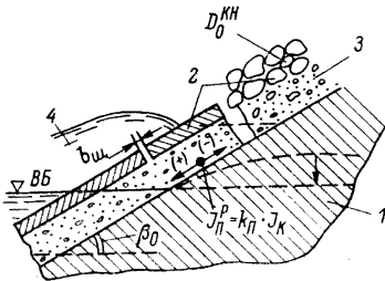
Рис. 34. К проектированию (подбору) фильтровой подготовки под крепления верхних откосов из связного (глинистого) грунта
