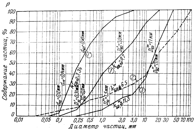
Рис. 12. Гранулометрический состав
