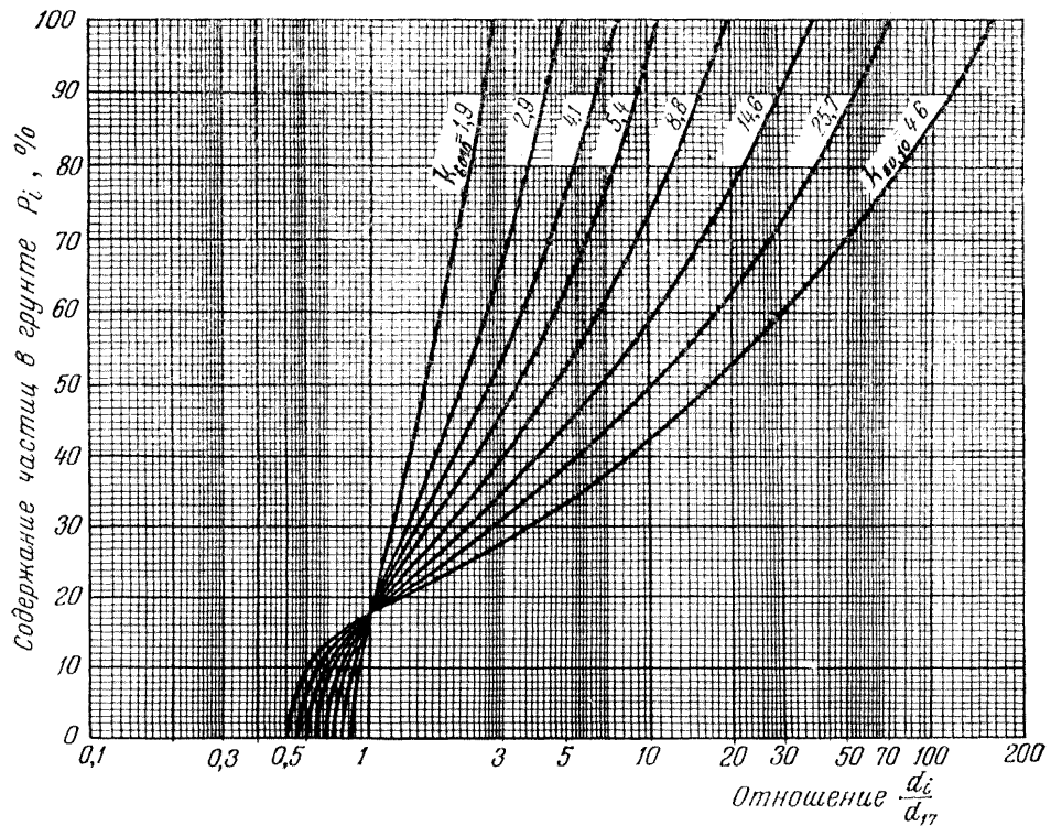
Рис. 2. Гранулометрический состав несuffозионных грунтов в относительных координатах.
