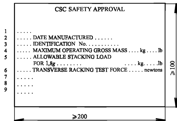
Рис. 4.1.2 Табличка КБК
