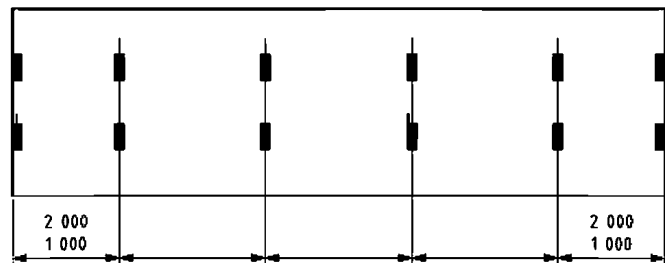
Рис. 2.3.2.5.1-2 Контактные площадки контейнеров 1BVB, 1BV, 1B и 1BX, имеющих 6 пар контактных площадок
