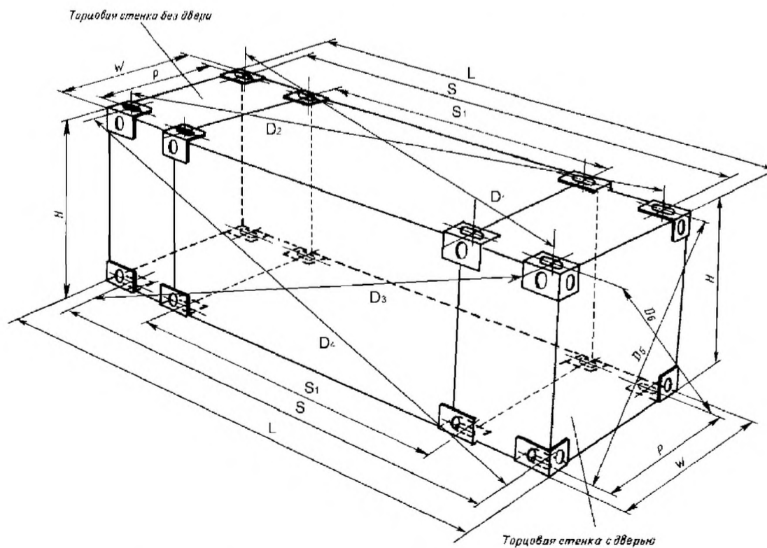
Рис. 2.2.1-6 Взаимное расположение фитингов в контейнерах 1EEE, 1EE.
