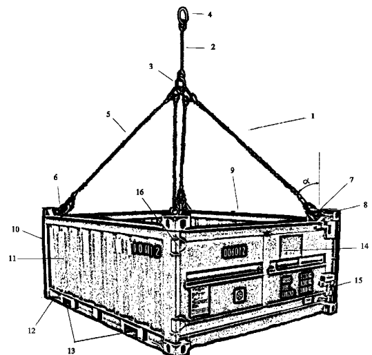
Рис. 1.2.1 Оффшорный контейнер:
