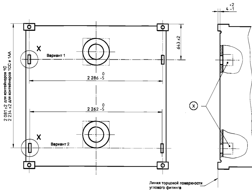
Вид X
