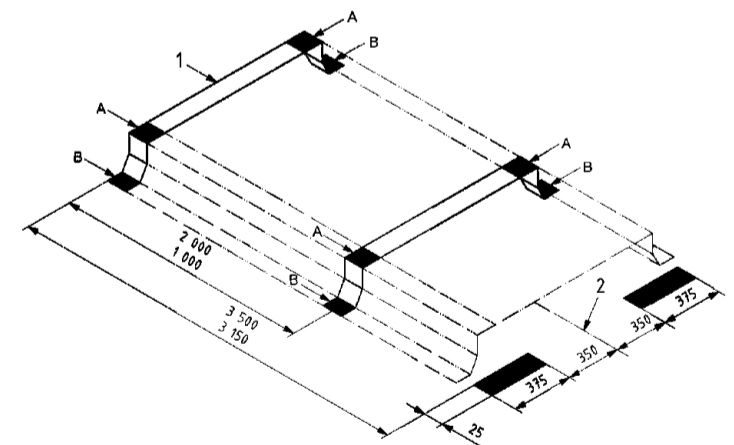
Рис. 2.3.2.5.2-4 Контактные площадки (контейнеры 1EEE, 1EE, 1AAA, 1AA, 1A и 1AX, имеющие паз «гусиная шея»): 1 — торец контейнера; 2 — центральная ось симметрии контейнера
