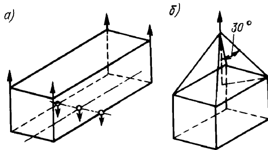
Рис. 3.2.3 Подъем за верхние угловые фитинги
