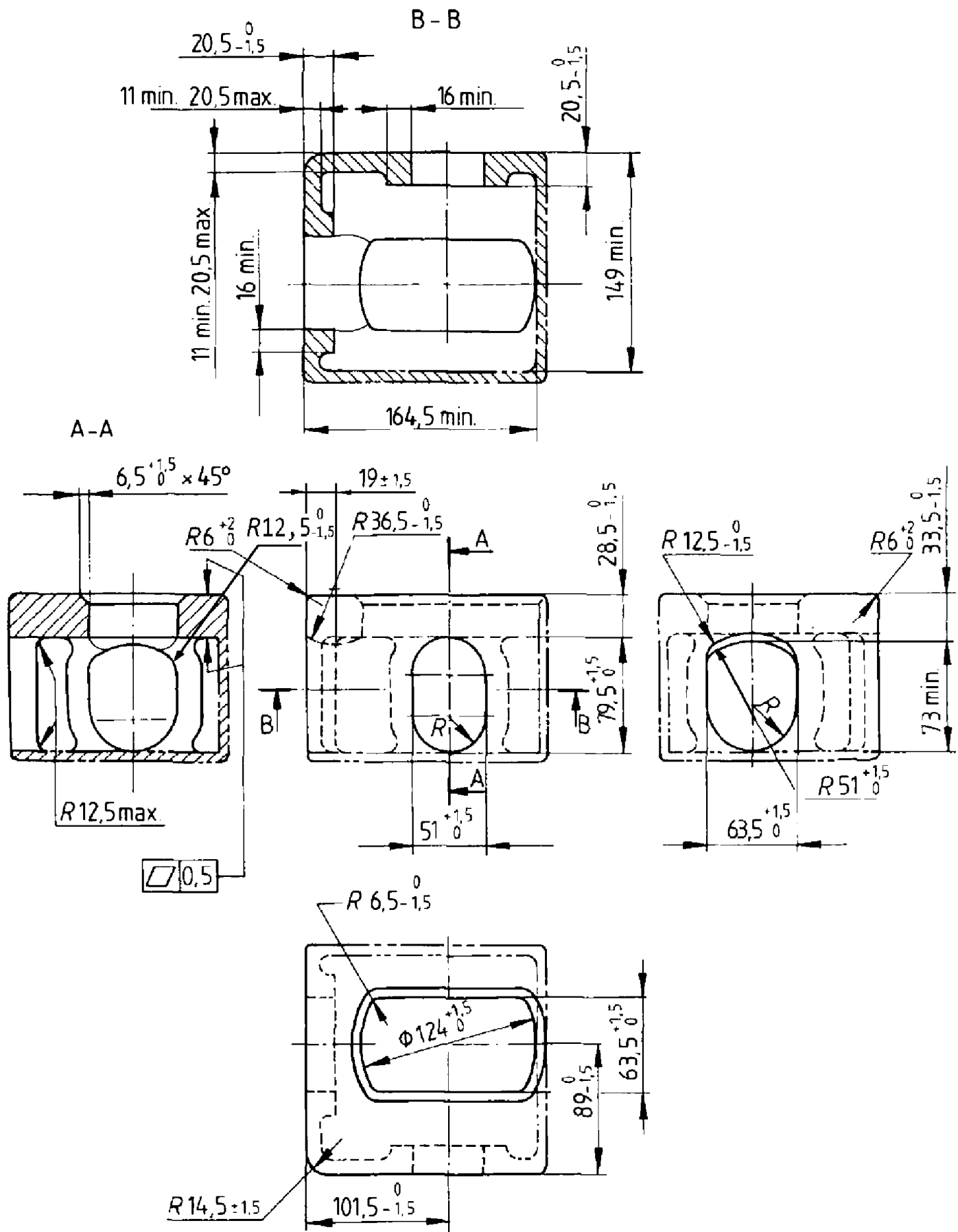
Рис. 2.2.1-1 Верхний угловой фитинг, мм:
