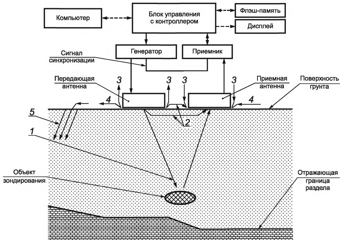
1 — зондирующий сигнал (объемная волна); 2 — сигнал прямого прохождения между антеннами; 3, 4 — сигналы, идущие в обратном и боковом направлениях; 5 — боковая волна, идущая в грунт
