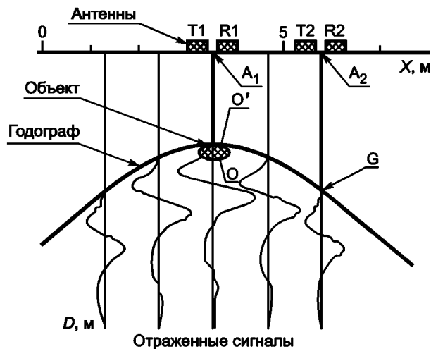
Расстояние |O'A_2| равно расстоянию |A_2G| по вертикали от центра антенного блока до точки G годографа. Вертикальная ось — глубина D
