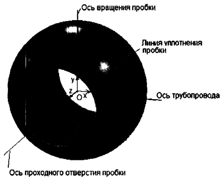
Рисунок 3 – Пробка шарового крана
