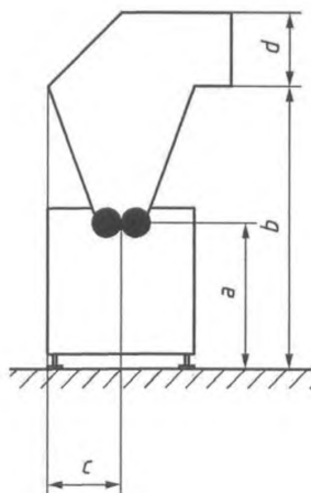
Рисунок 11 — Питающий бункер с воротниковой воронкой
