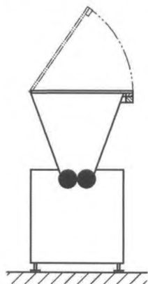
Рисунок 5 — Жесткое защитное ограждение с блокирующим устройством
