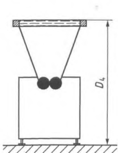
Рисунок 12 — Загрузочный бункер с электрочувствительным защитным оборудованием (ESPE)
