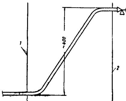
Рис. 10. Вывод трубок из ко- жуха к тепловым вентилям 1 — кожух внутренний; 2 — кожух наружный
