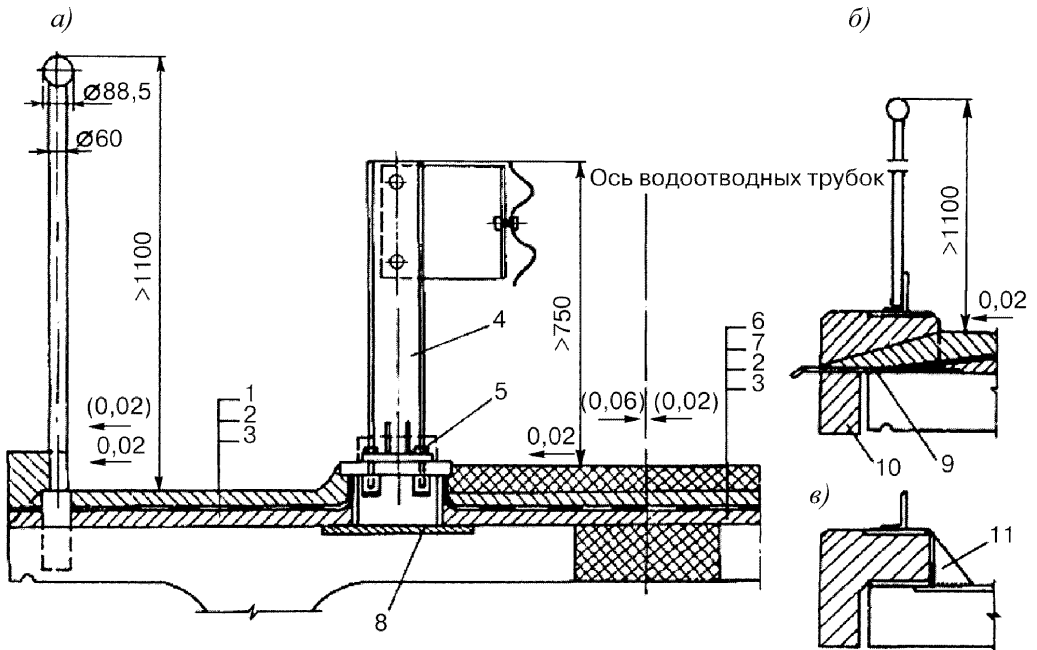
а) – без карнизного блока; б) – с карнизным блоком; в) – крепление карнизного блока (в скобках приведены значения при водоотводе через трубки);
