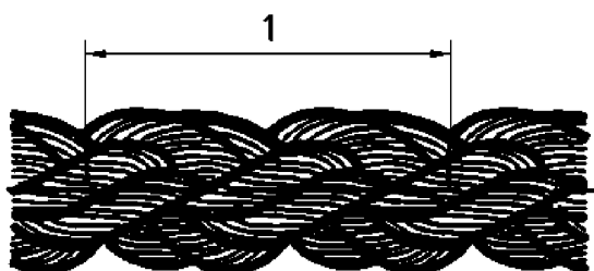
1 — один шаг плетения
