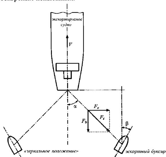
Рис. 2.1.2 Типовая схема эскортных операций:
