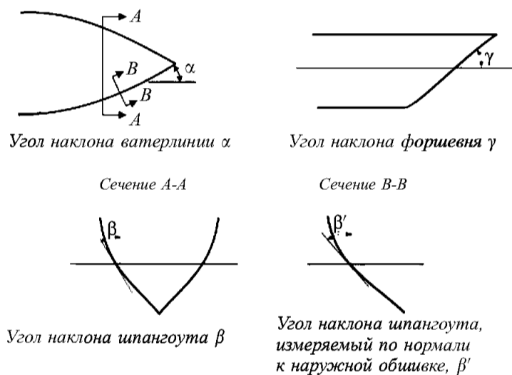
Рис. 1.2.3.2.1.1.1 Определение углов наклона
