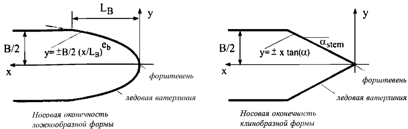
Рис. 1.2.13.2.1-1 Определение формы носовой оконечности
