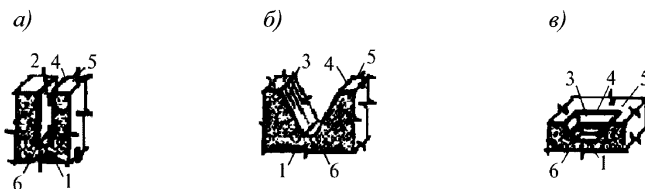
а), б) – траншеи с прямыми боковыми стенками и с откосами; в) – котлован 1 – дно; 2 – боковая стенка; 3 – боковой откос; 4 – бровка; 5 – берма; 6 – подошва
