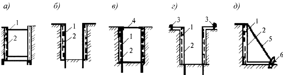
а) – распорное; б) – консольное; в) – консольно-распорное; г) – консольно-анкерное; д) – подкосное; 1 – шиты; 2 – стойки (сваи); 3 – анкера; 4 – распорки; 5 – подкосы; 6 – упоры
