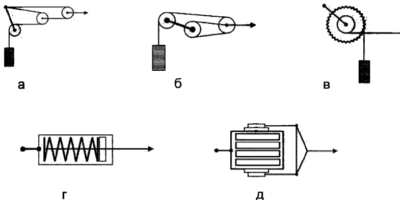
а — блочный; б — блочно-полиспластный; в — барабанный; г — пружинный с продольным расположением пружин; д — пружинный с поперечным расположением пружин
