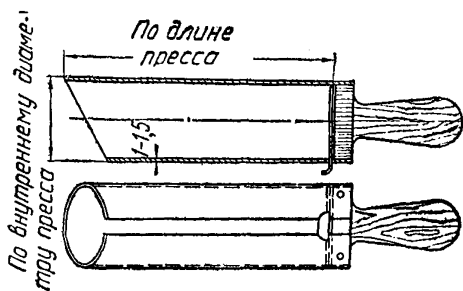
Рис. 11. Совок для наполнения шприца
