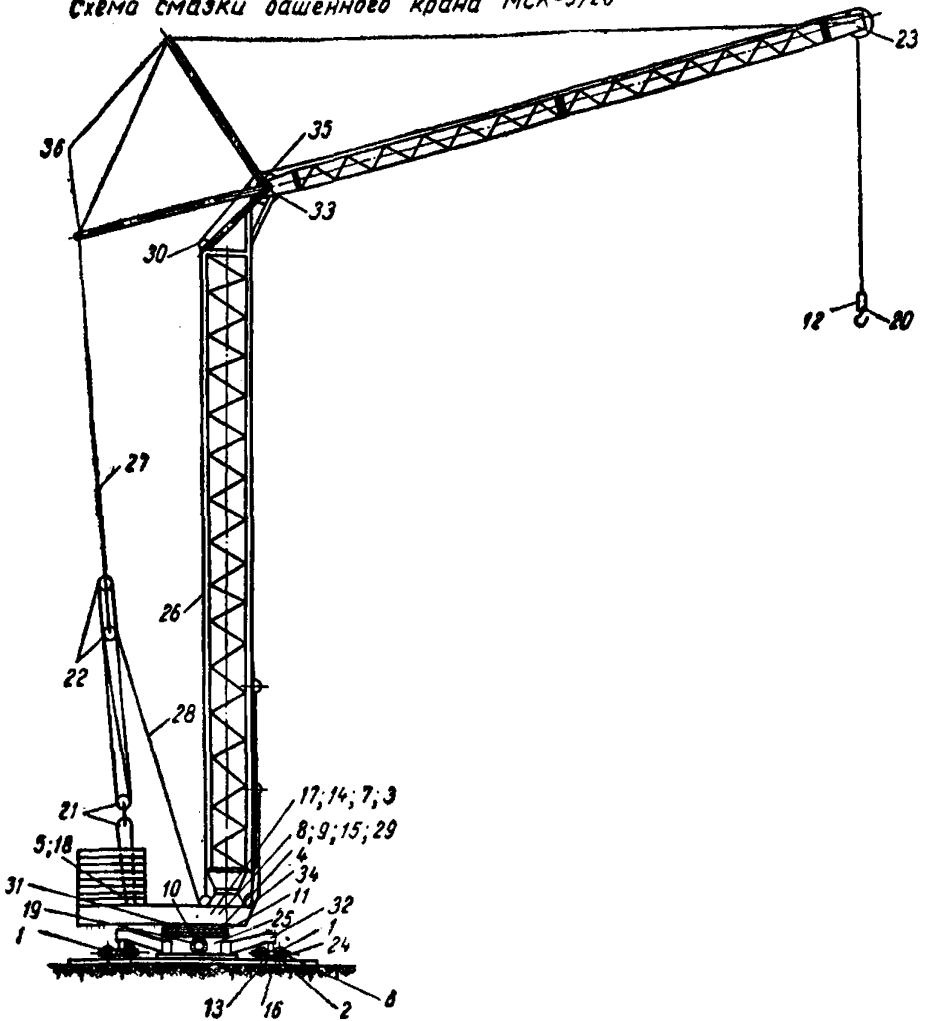
Смазка башенного крана МСК-5/20
