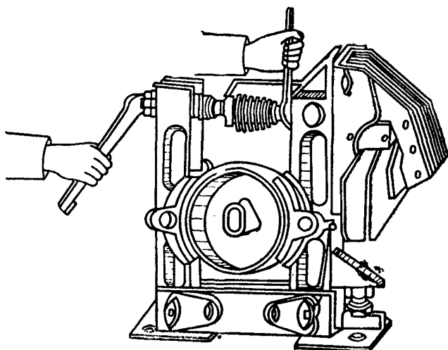
Рис. 28. Раздвижение рычагов «отжимной гайкой»
