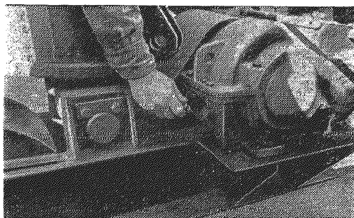
Рис. 2. Проверка уровня масла маслостерной линейкой в корпусе редуктора механизма передвижения башенного крана МСК-5/20
