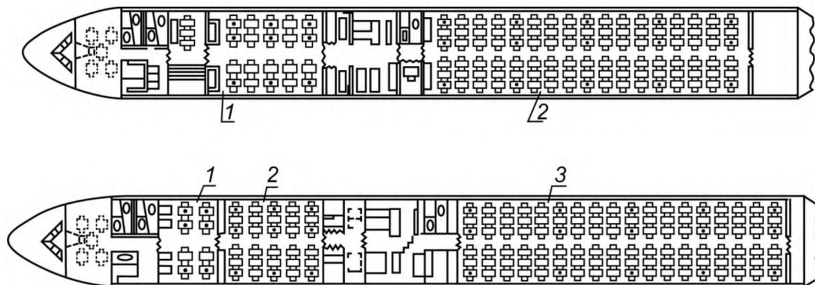
1 – салон первого класса, 2 – салон туристского класса, 3 – салон туристского и экономического классов
