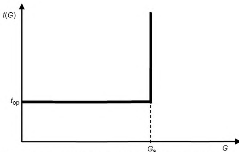
Рисунок 3 — Независимая характеристика времени реле недостаточного напряжения
