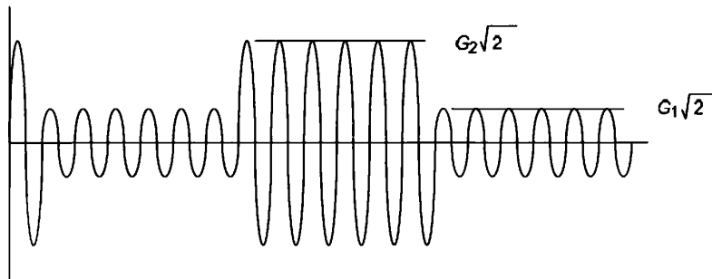
Рисунок 12 — Испытательная осциллограмма
