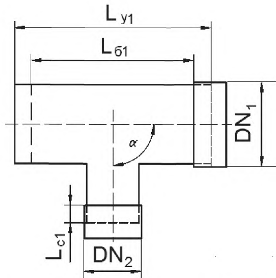
Рисунок А.7 – Неравнопроходной (переходной) тройник
