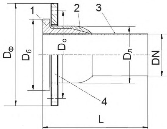
Рисунок А.8 –Фиксированный фланец
