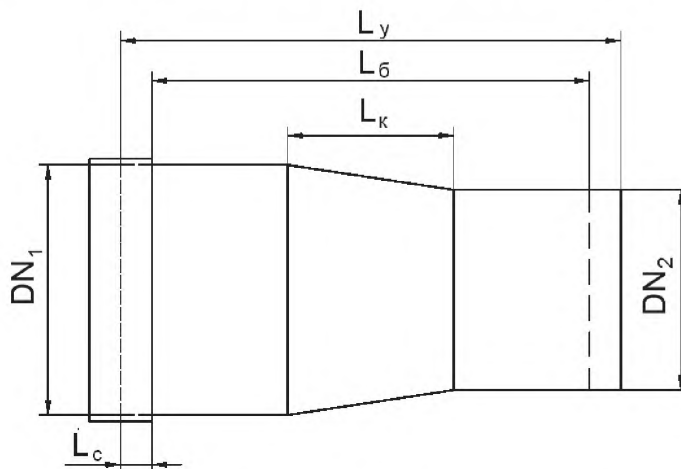
Рисунок А.4 – Концентрический переход
