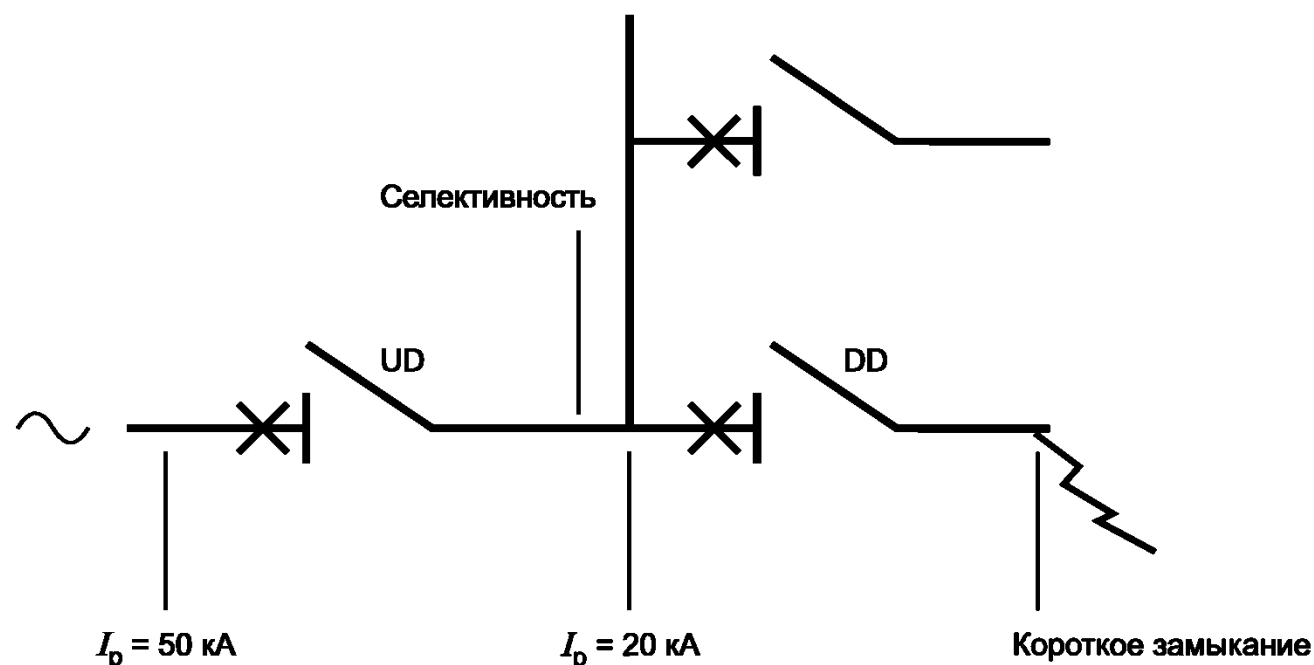
Рисунок А.4 — Пример координации автоматических выключателей с максимальным уровнем тока короткого замыкания 50 кА и уровнем тока повреждения 20 кА
