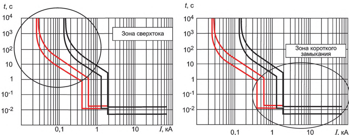
Рисунок В.1 — Зоны сверхтоков и короткого замыкания
