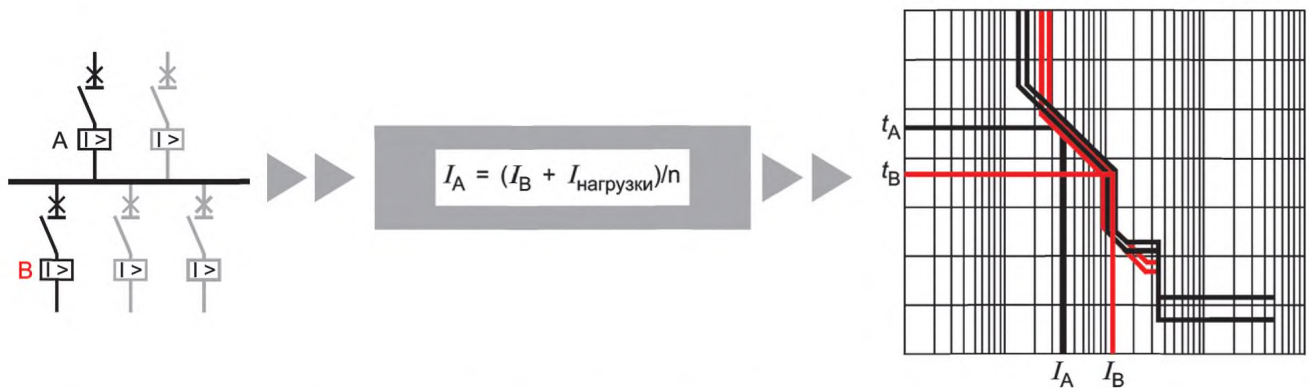
Рисунок В.2b — Последовательно включенные УТЗ (ОСПД), несколько нагрузок (разветвляющийся ток)
