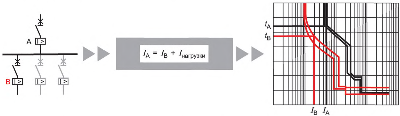
Рисунок В.2b — Последовательно включенные УТЗ (ОСПД), несколько нагрузок (разветвляющийся ток)
