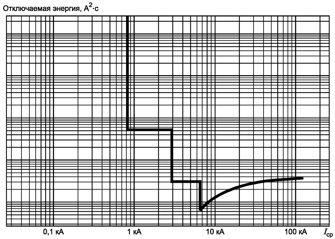
Рисунок 2 — Пример характеристики интеграла Джоуля ( I^2t ) автоматического выключателя
