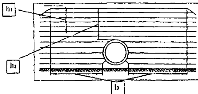
К.4 Засыпка бетонных и железобетонных водопропускных труб.
