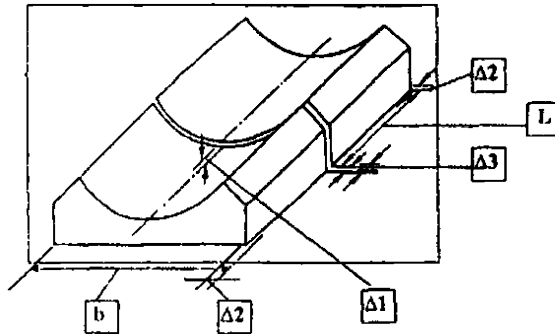
Рисунок К.1 – Конструкция сборного фундамента из лекальных блоков
