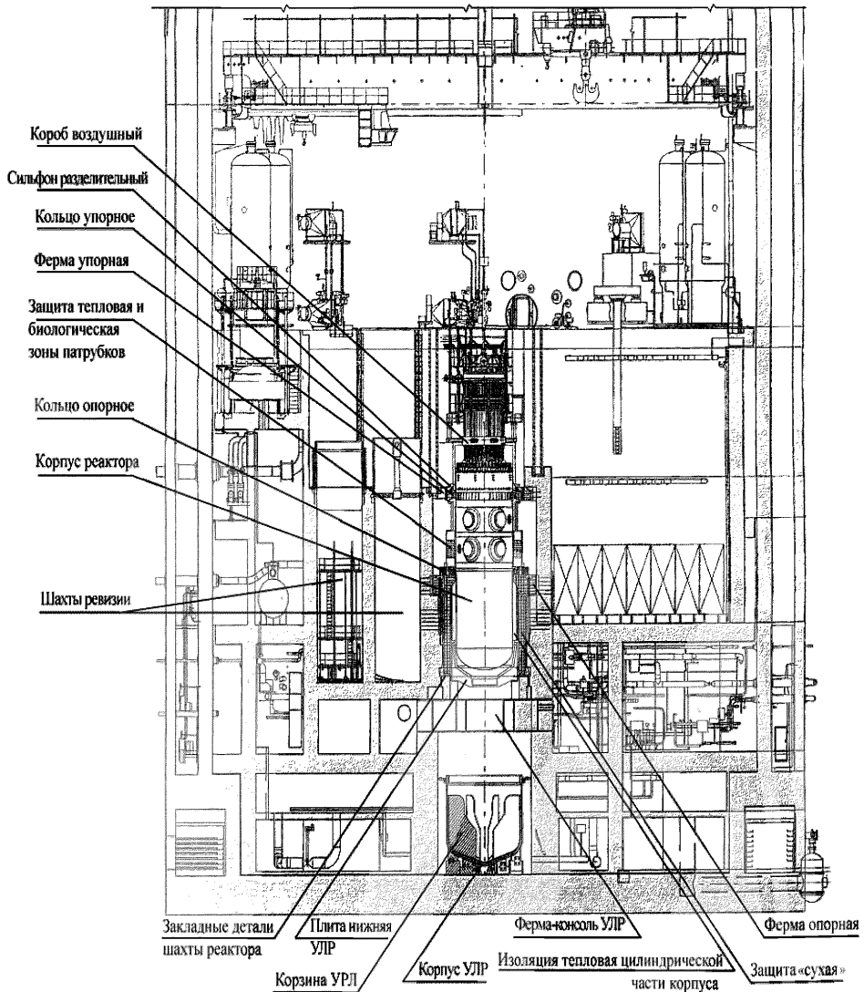
Рисунок 1 – Оборудование шахты реактора
