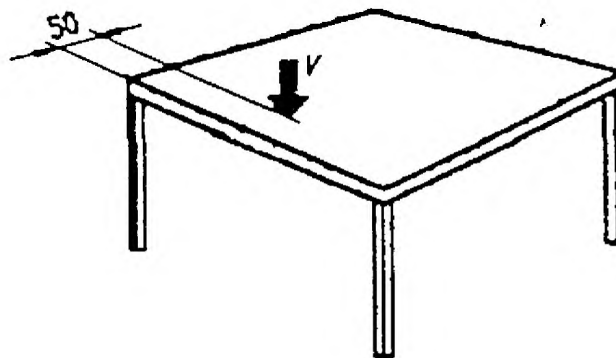
Рисунок 7 – Испытание на устойчивость под действием вертикальной нагрузки
