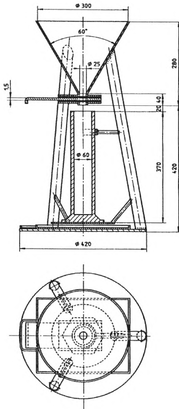
Рисунок 1 – Аппарат для определения насыпной плотности удобрений без уплотнения
