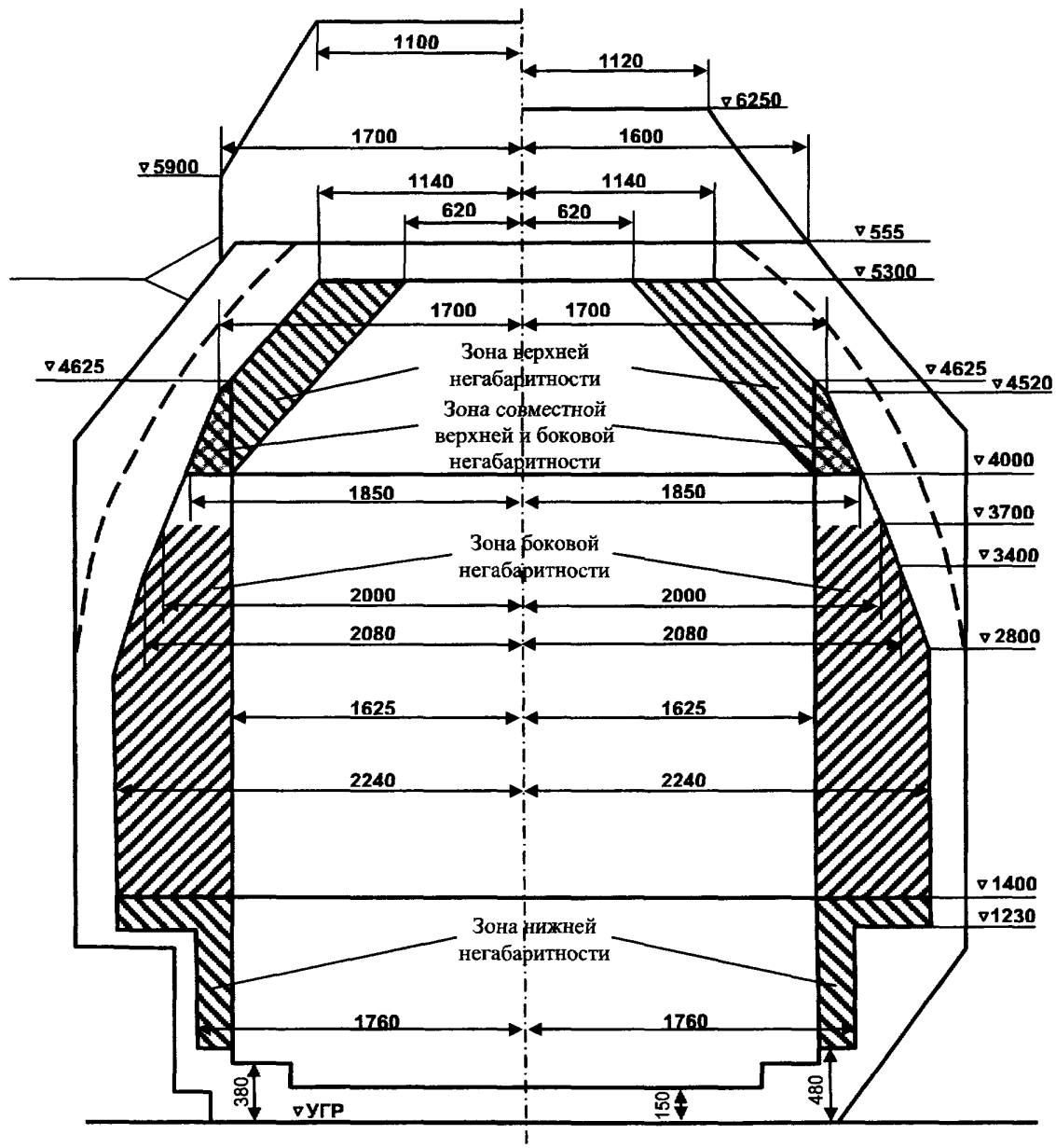
Рис.1. Зоны негабаритности груза
