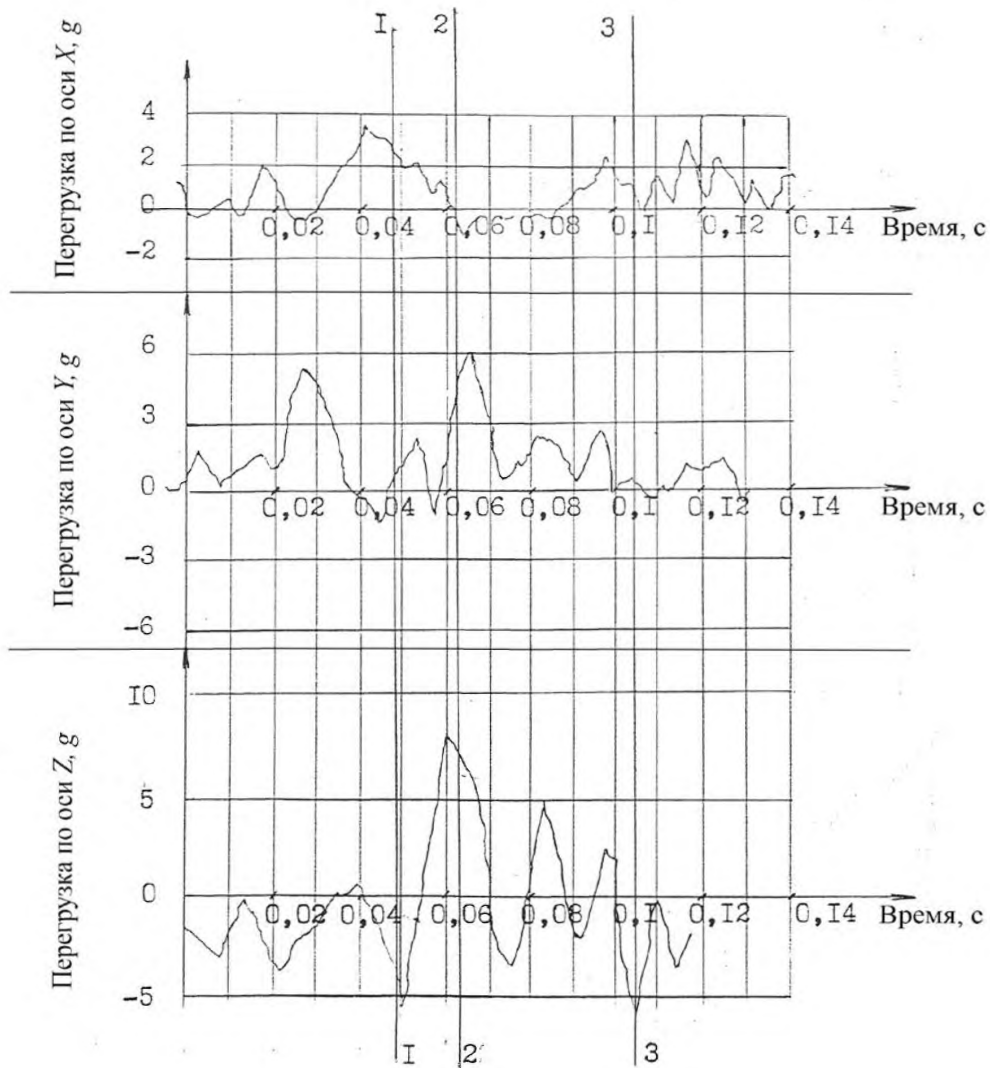
1, 2, 3 — сечения с максимальными перегрузками по осям X, Y и Z
