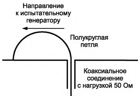
Рисунок D.3 – Полуциркулярная петля на пластине заземления
