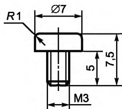
Симметрично вращающаяся часть Верхняя часть центрального проводника. Нержавеющая сталь. Приблизительно 2:1
