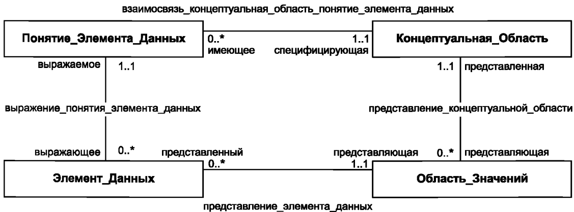
Рисунок 3 — Общий вид метамодели
