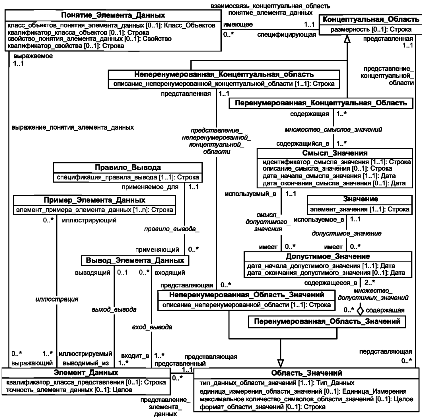
Рисунок 11 — Консолидированная метамодель
