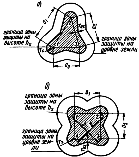
Рис. 15. Зона защиты многократного стержневого молниеотвода
