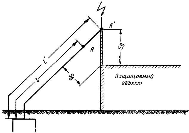
Рис. 4. Стержневой молниевод, изолированный от защищаемого объекта деревянной стойкой
