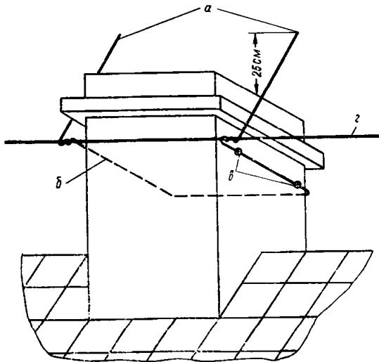
Рис. 27. Крепление молниеприемника к дымовой трубе а — вилка; б — вязальная проволока; в — скобка; з — молниеприемник
