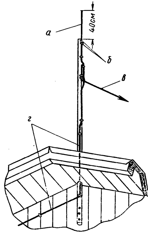
Рис. 26. Молниезащита при плоской крыше а — стержневой молниеприемник; б — скобка; в — тросовый молниеприемник; з — токоотвод
