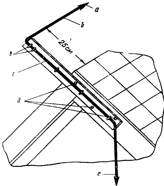
Рис. 25. Молниезащита при крутой крыше а — к дымовой трубе; б — молниеприемник; в — скобка; з — доска; д — гвозди; е — токоотвод
