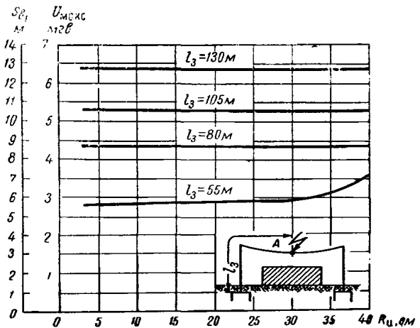
Рис. 6. Потенциал в средней точке тросового молниеотвода при ударе молнии в середине пролета
