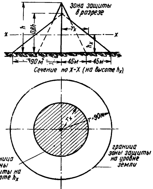
Рис. 12. Зона защиты одиночного стержневого молниеотвода высотой от 60 до 100 м
