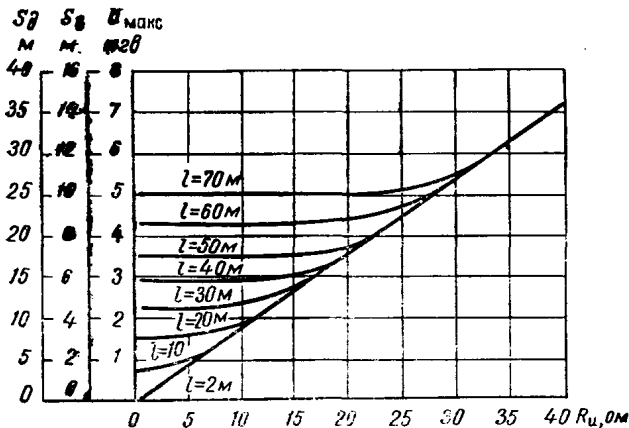
Рис. 5. Максимальный потенциал стержневого молниеотвода на высоте $l(l')$
