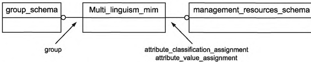
Рисунок D.1 — Представление ИММ на уровне схем в формате EXPRESS-G (диаграмма 1 из 1)
