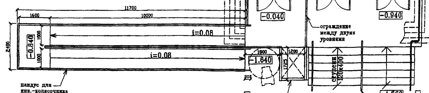
Фрагмент плана по главному входу
