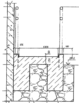
Разрез пандуса
