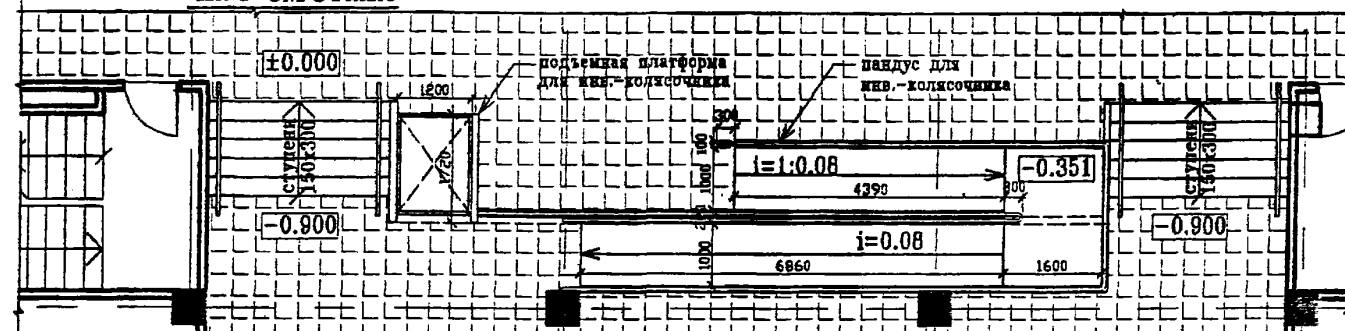
Фрагмент плана вестибюля с пандусом и платформой
