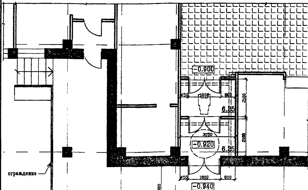
Фрагмент плана балкона-пожаростойника на 3-ом этаже
