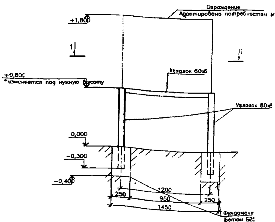
Пример ТОЭ 3.
