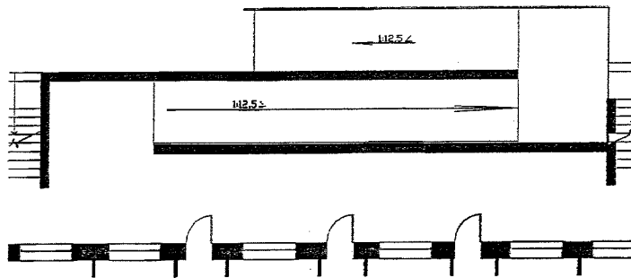
Организация пандуса с внутренней стороны поликлиники
