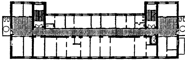
План 2-го и 3-го этажей
