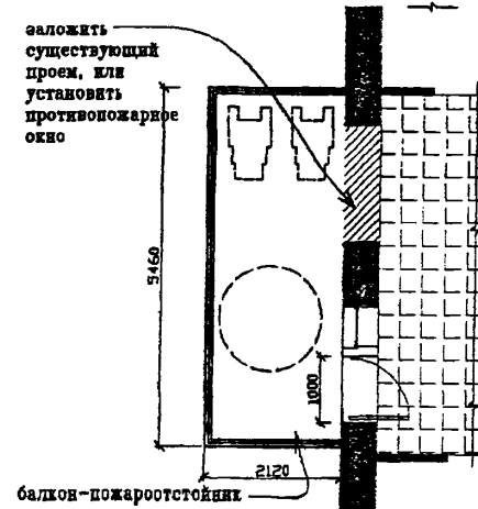
Фрагмент плана балкона-пожаростойника на 3-ом и 4-ом этажах
