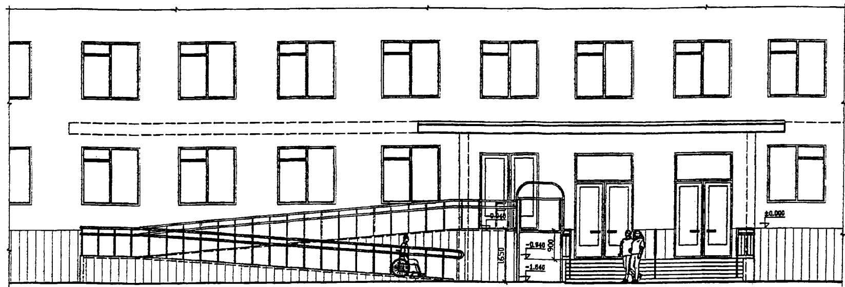
Фрагмент фасада по главному входу
