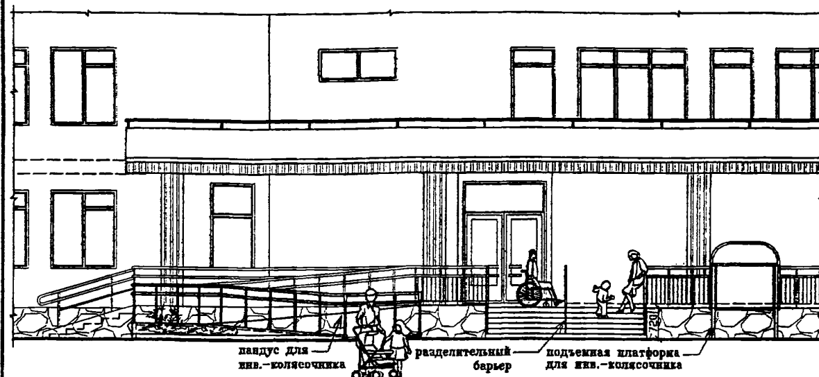
Фрагмент фасада по входу
