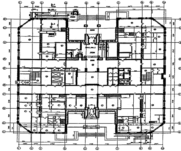
План 1 этажа
