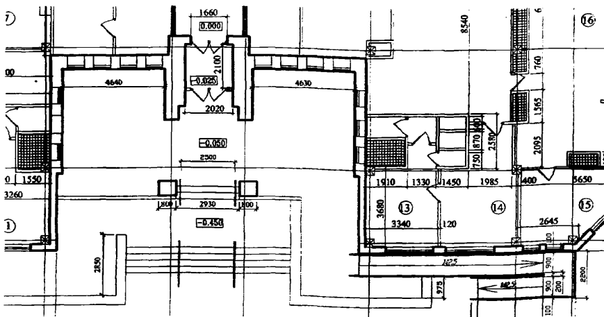
План входной зоны со стороны детского отделения
