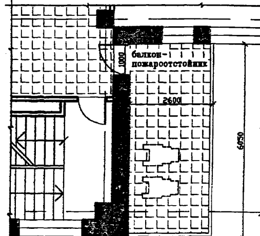
Фрагмент плана балкона-пожаростойника на 3-ом этаже
