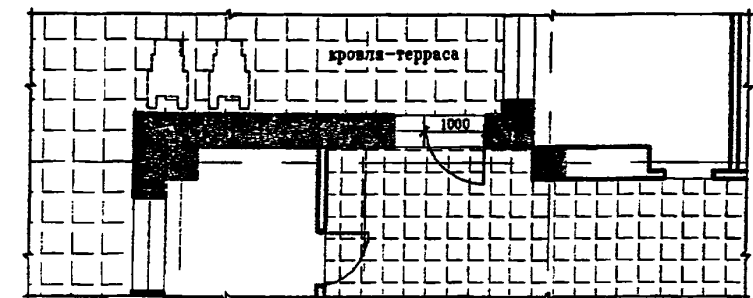
Фрагмент плана с выходом на кровлю - террасу на 4-ом этаже
