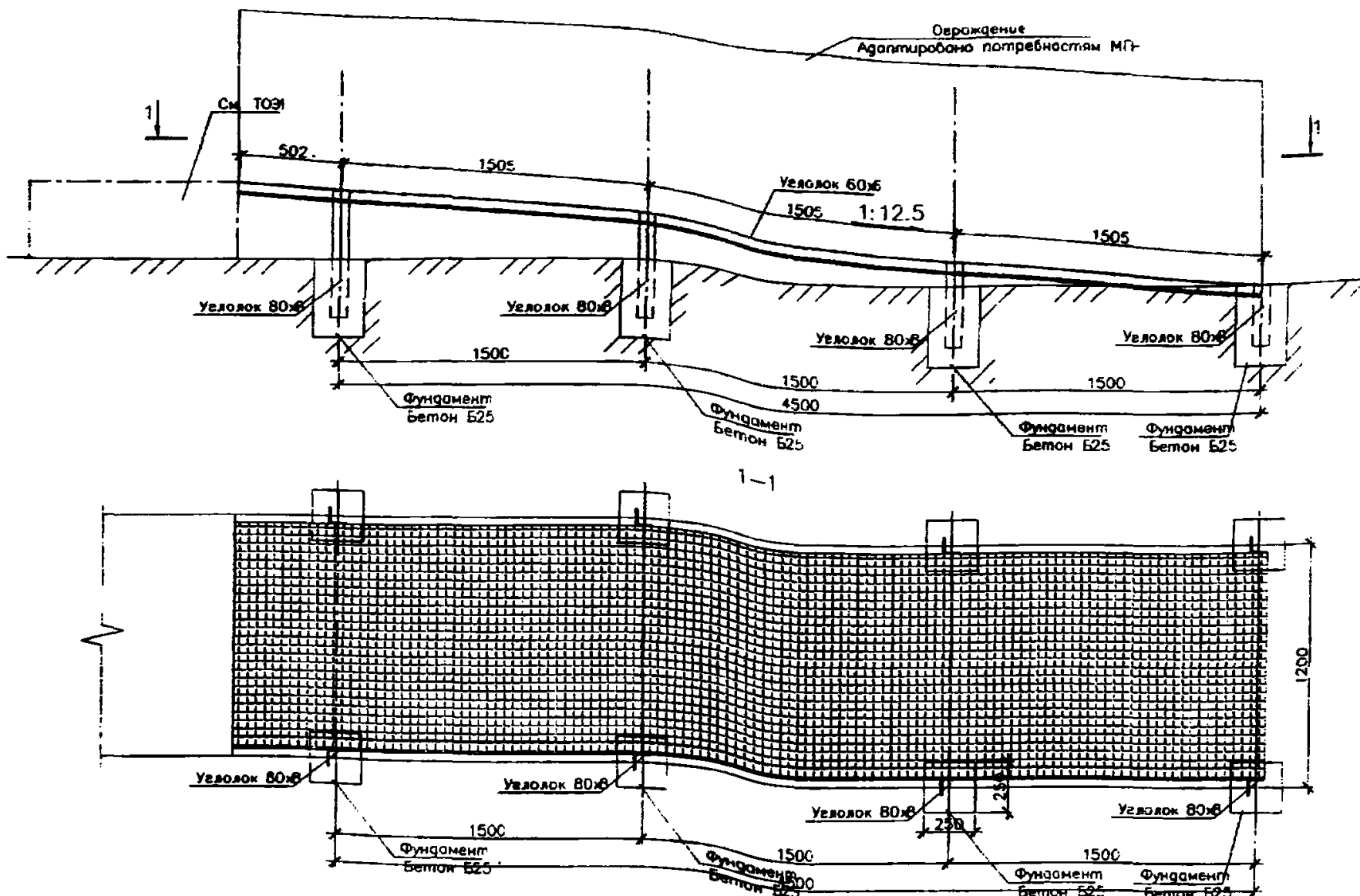
Пример ТОЭ 2.
