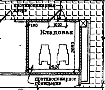
Противопожарное помещение на 4-ом этаже
