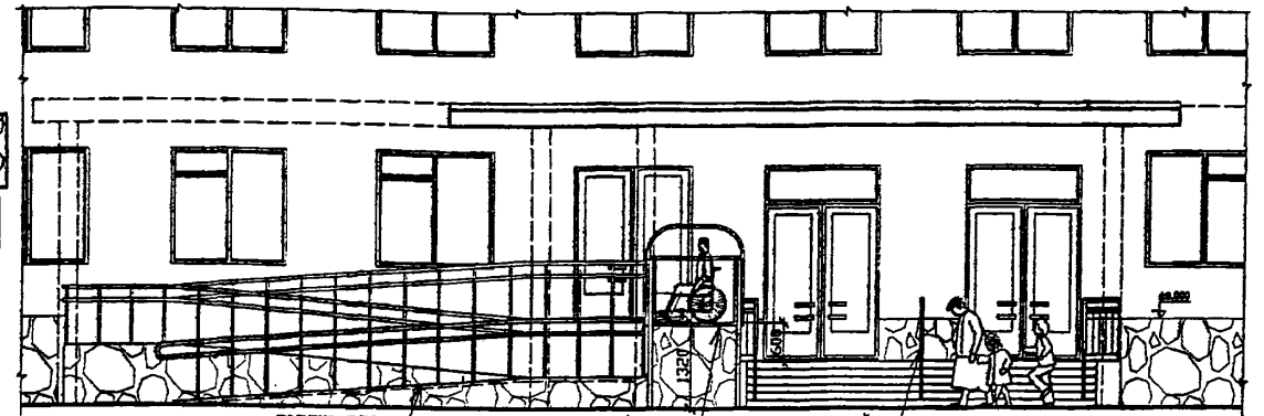
пантус для инв.-колясочника, подъемная платформа для инв.-колясочника, разделительный барьер Фрагмент фасада по главному входу
