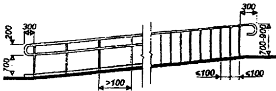
Схемы расположения поручней пандусов (по СП 35-101)
