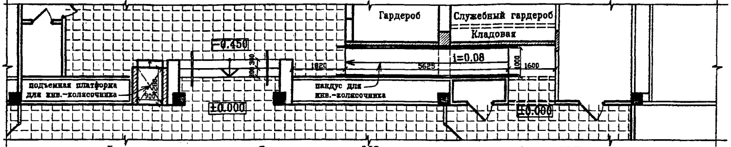
Фрагмент плана вестибюля по входу N2
