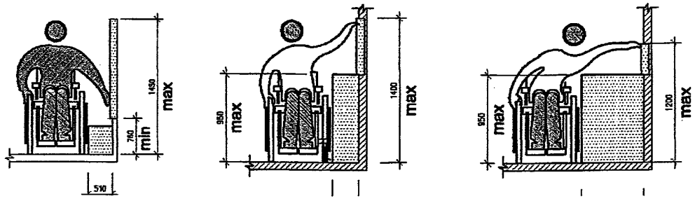
Параметры фронтальной досягаемости человека на кресле-коляске
