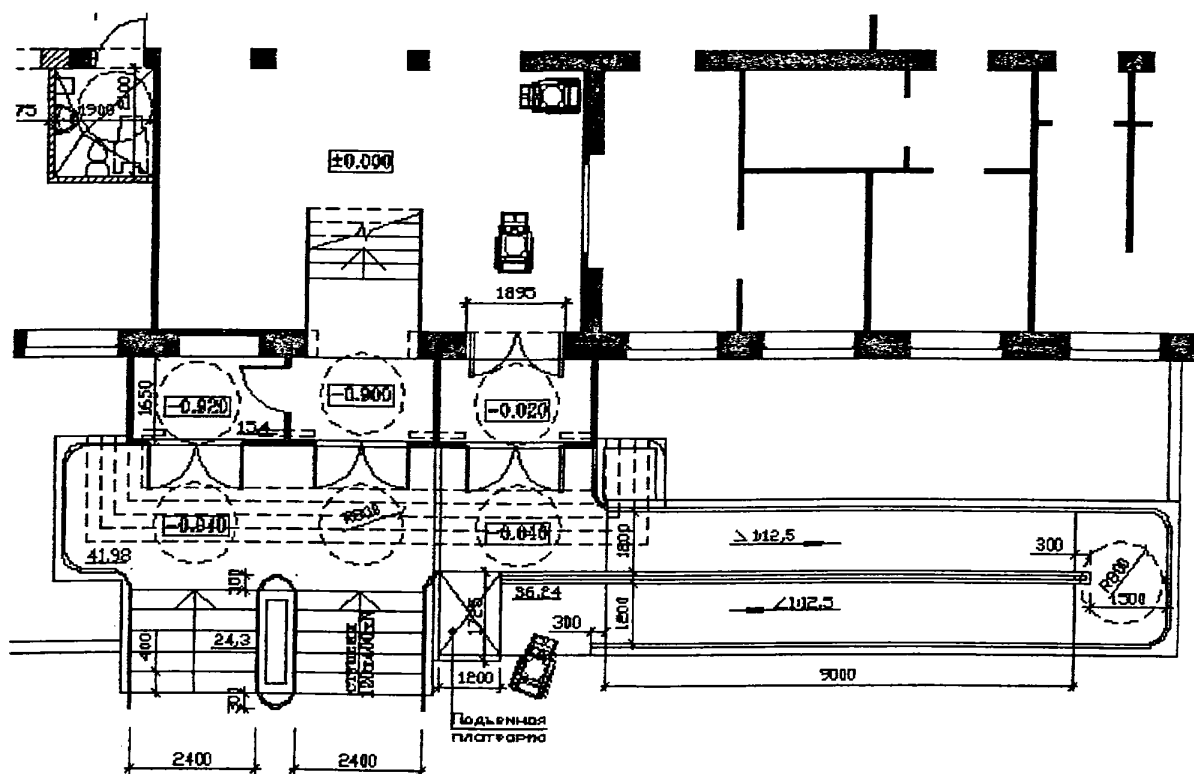
Фрагмент плана главного входа с включением элементов доступности МГН
