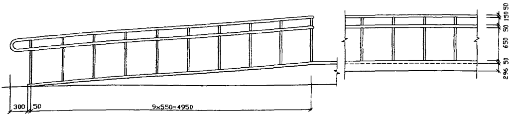
Ограждение пандуса
