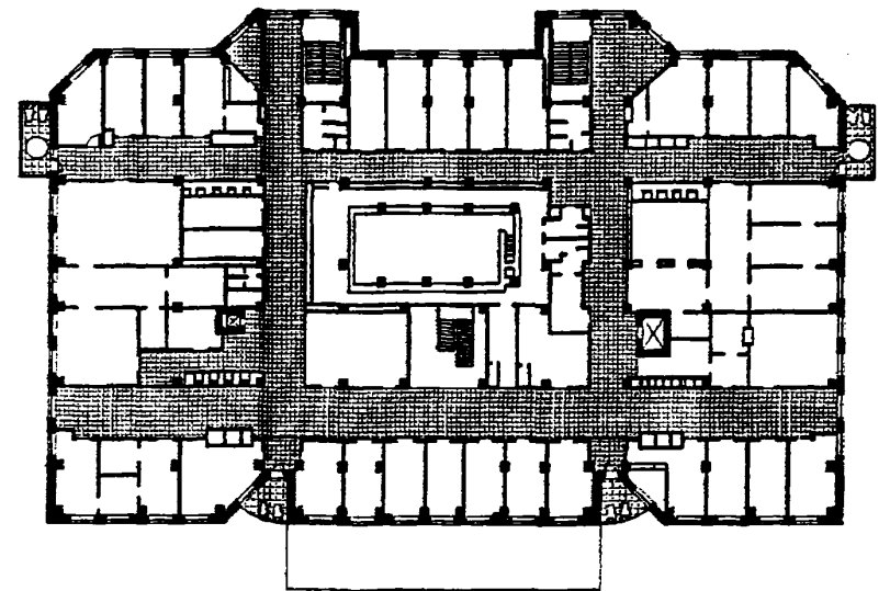
План 2-го и 3-го этажей
