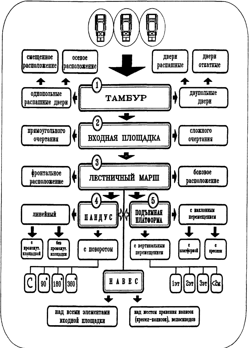
Функционально-типологическая схема входного узла
