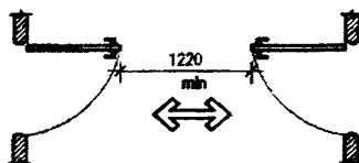
4. Минимальное расстояние между открывающимися дверными проемами при внутреннем (встречном) открывании
