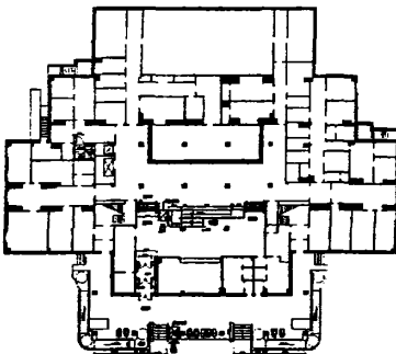
План 1 этажа
