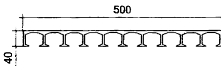
Сечение настольной панели с износостойким покрытием из стеклопластикового пулпрузионного профиля (возможен подогрев)
