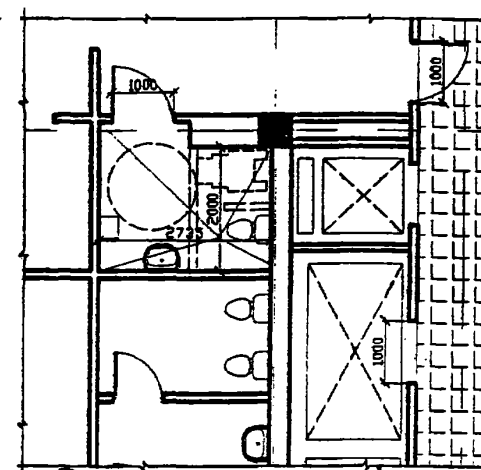
Фрагмент плана с лифтом и туалетом на 1-ом этаже
