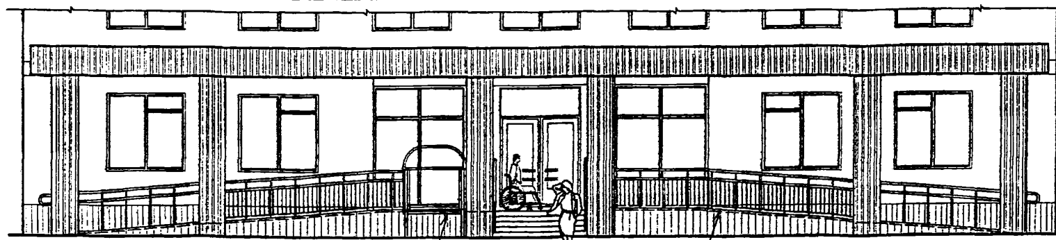
Фрагмент фасада по входу
