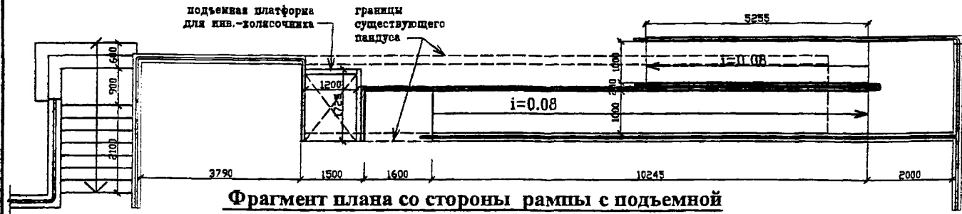
План 1-го этажа
