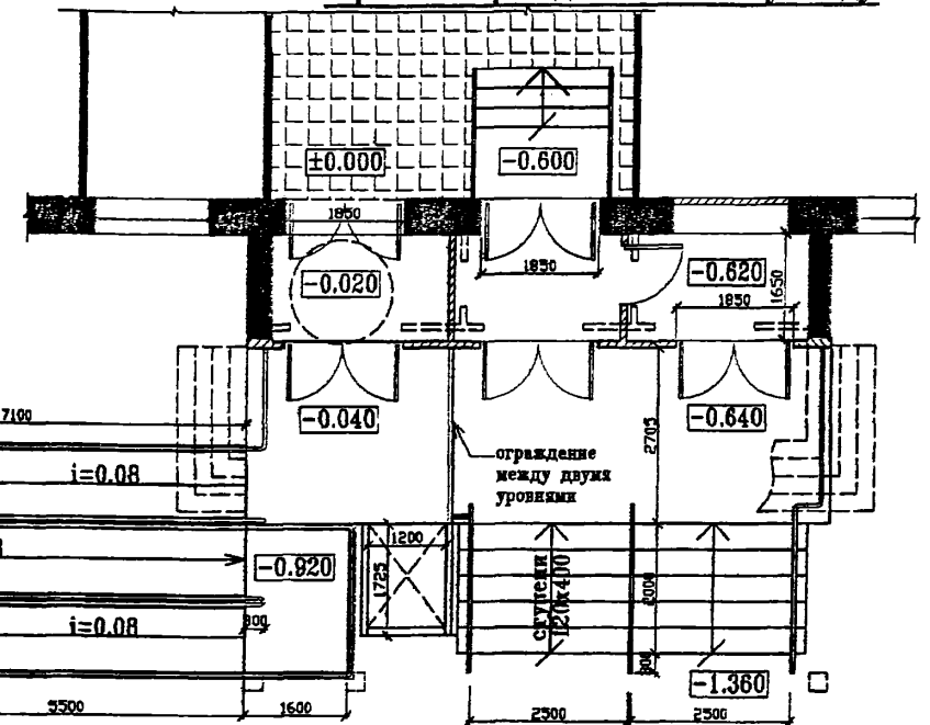
Фрагмент плана по главному входу
