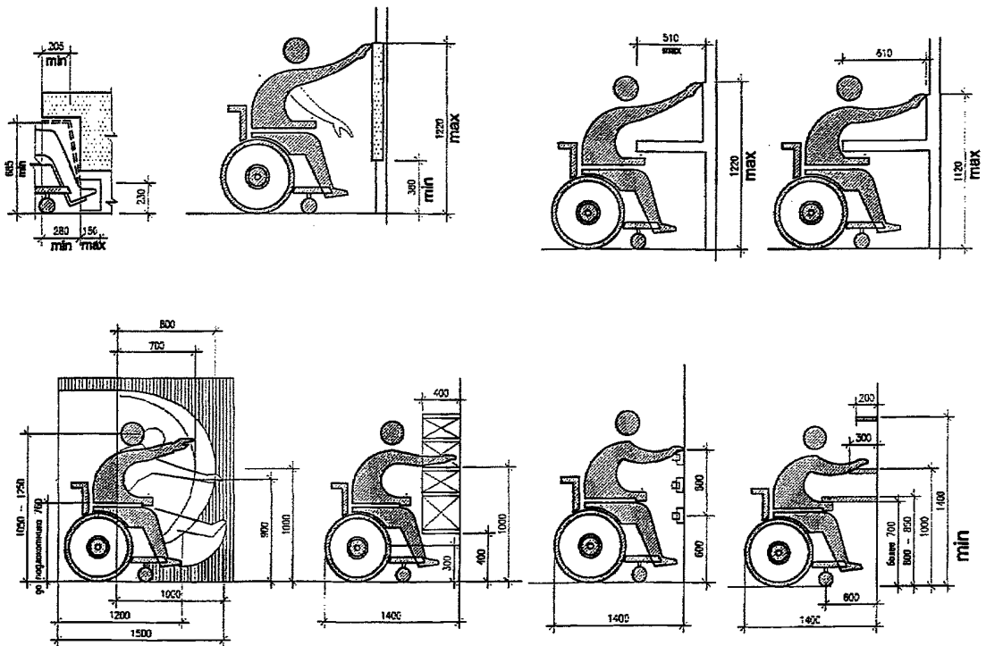
Параметры фронтальной досягаемости человека на кресле-коляске
