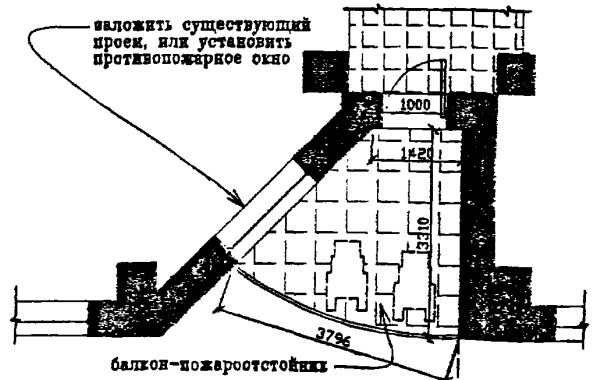
Фрагмент плана балкона на 2-ом и 3-ом этажах
