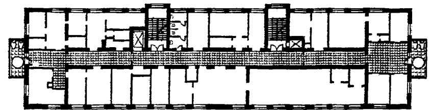
Plan типового этажа
