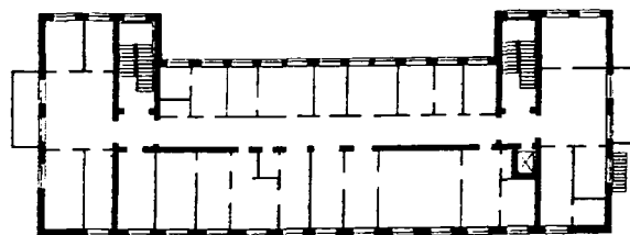
План 2 этажа
