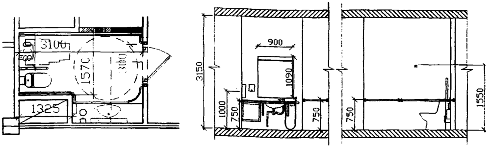
План реконструкции поэтажного санитарного узла для инвалида-колясочника
