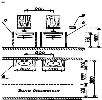
Зона расположения инвалидной коляски около умывальника (по 3.10 СП-35-101)
