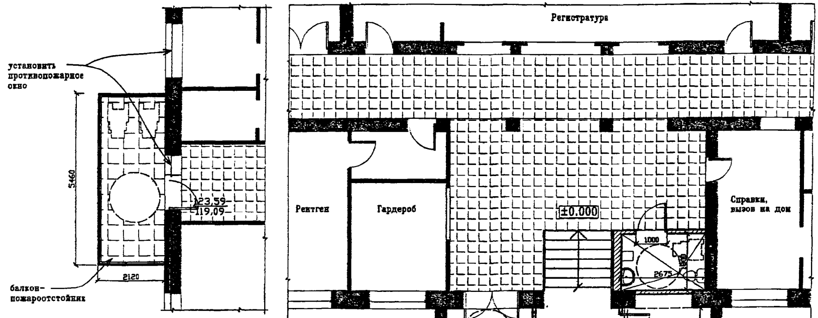
Фрагмент плана балкона-пожаростойника на типовых этажах
