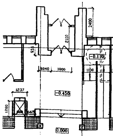
План вестибюля с внутренним пандусом и подъемной платформой
