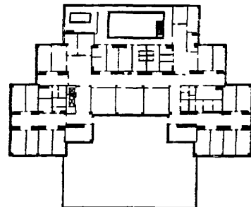
План 3 этажа
