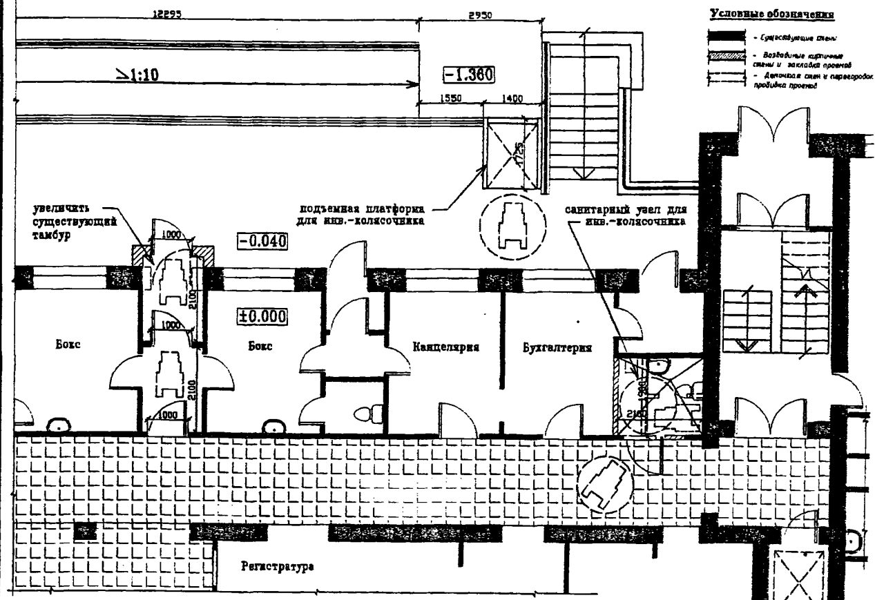
Фрагмент плана со стороны рампы с подъемной платформой, сан. узлом и лифтом
