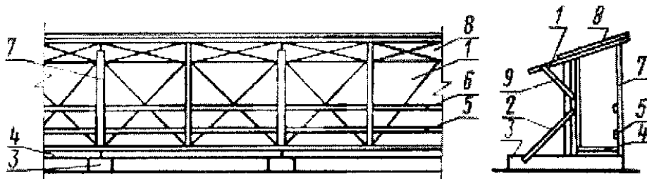
г) ограждения с детальными элементами
