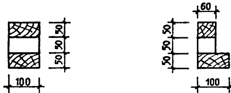
Рис. П.4.3. Сечения стоек каркаса.
