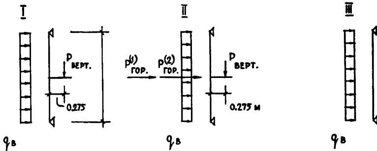
Рис. П.4.4. Возможные сочетания нагрузок
