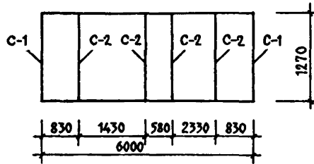
Рис. П.4.2. Схема каркаса
