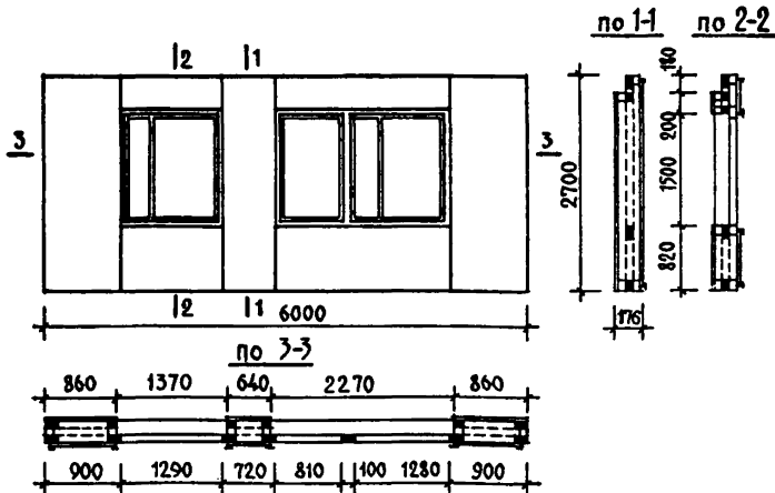
Рис. П.4.1. Общий вид и разрез панели
