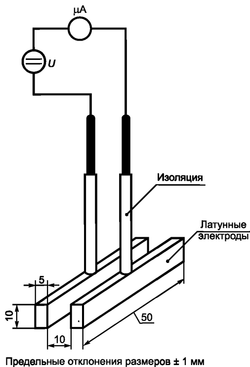
Рисунок 1 — Испытательная установка для определения диэлектрических свойств заполнителя
