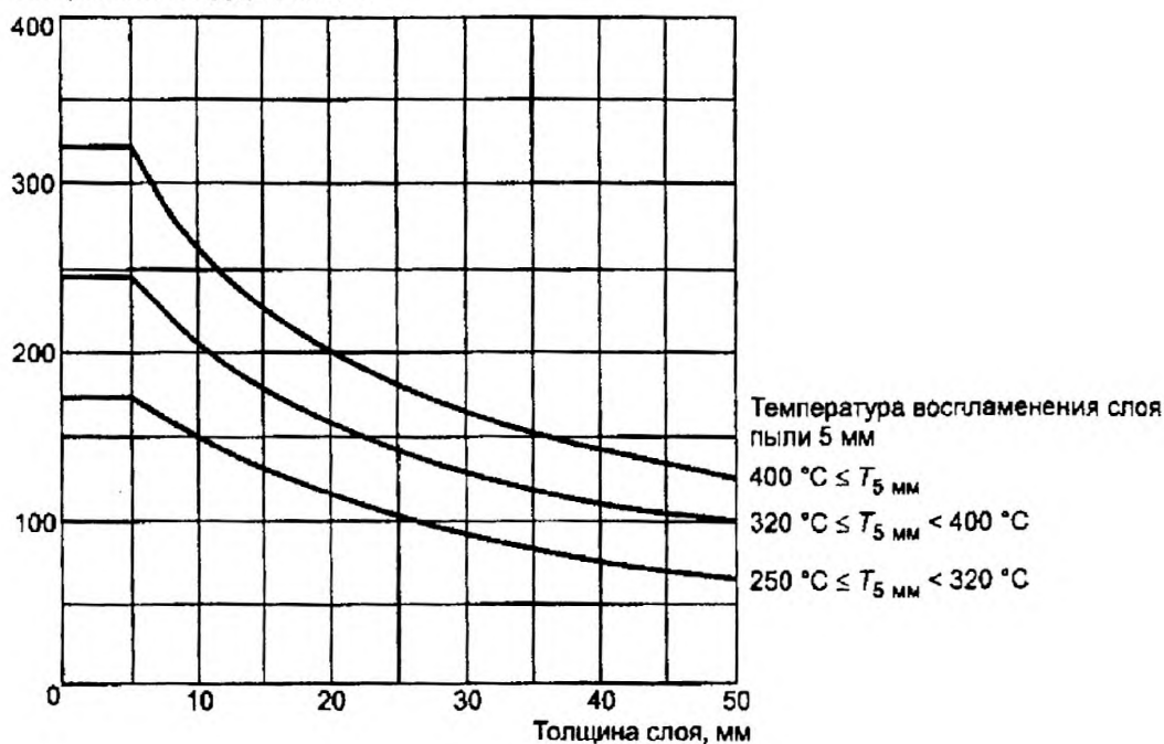
Максимальная допустимая температура поверхности оборудования, °С
