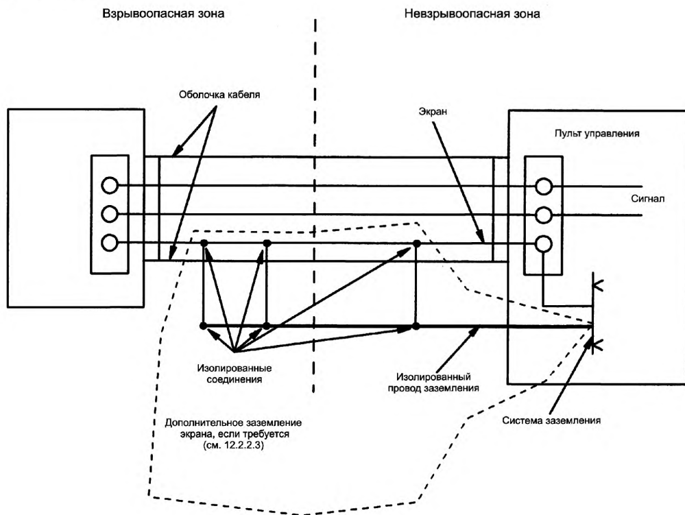
Рисунок 2 - Заземление проводящих экранов
