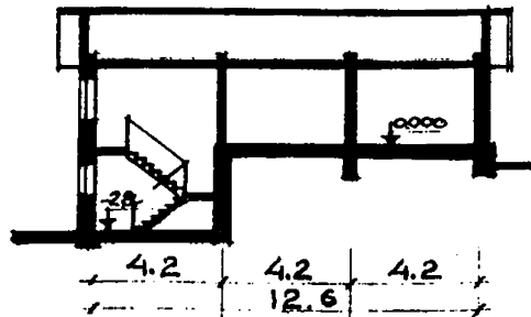
РАЗРЕЗ
