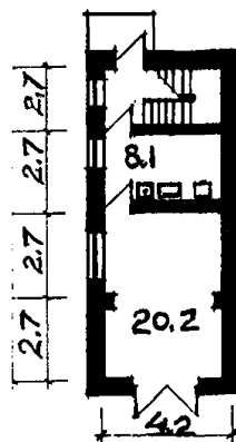
ПЛАН ЦОКОЛЬНОГО ЭТАЖА
