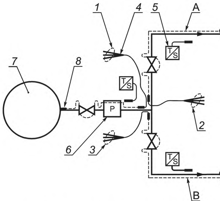
A — труба А; B — труба В; 1 — цепь № 1; 2 — цепь № 2; 3 — цепь № 3; 4 — заделка холодного конца; 5 — температурный датчик; 6 — насос; 7 — обогреваемый резервуар; 8 — заделка горячего конца
