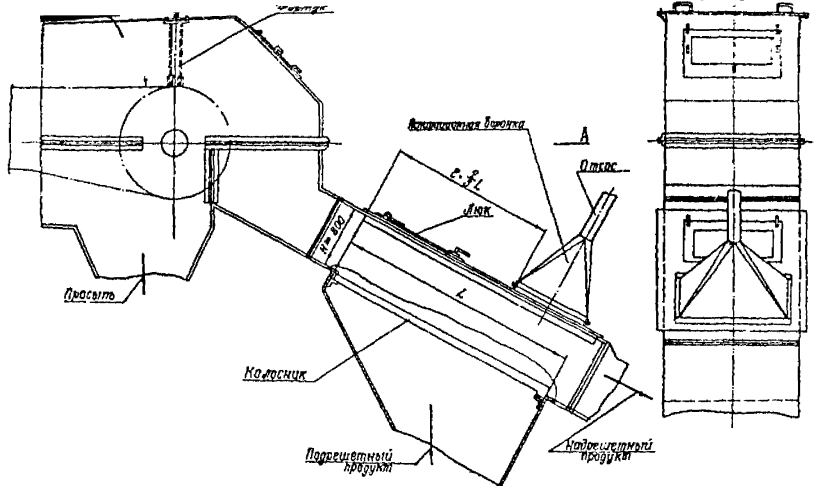
Укрытие неподвижного колосникового прохода
