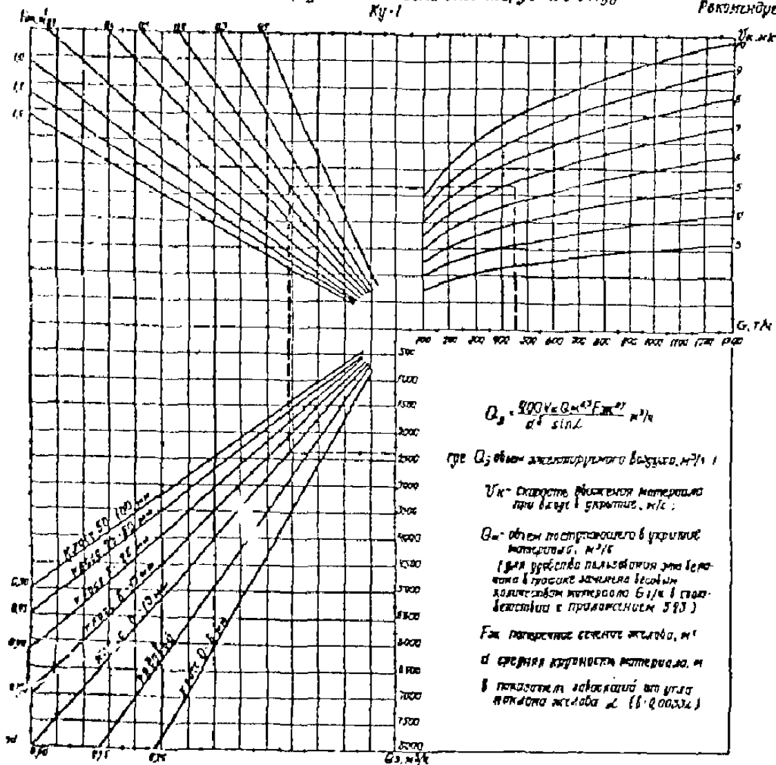
График для определения объема эжектируемого воздуха Ky-1
