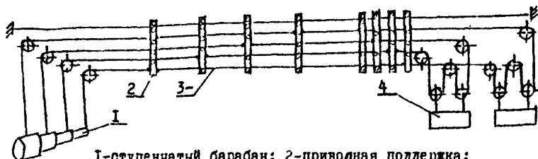
1-ступенчатый барабан; 2-приводная поддержка; 3-тяговый канат для передвижения поддержек; 4-полиспасное натяжное устройство
