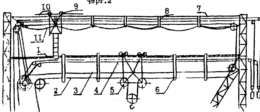
1-несущий канат; 2-подъемный канат; 3-тяговый канат для передвижения грузовой тележки; 4-тяговый канат для передвижения поддержки; 5-грузовая тележка; 6-поддержка приводная; 8-неподвижная закрытая поддержка; 9-ремонтная тележка; 10-тяговый канат для передвижения ремонтной тележки; II-электротележка
