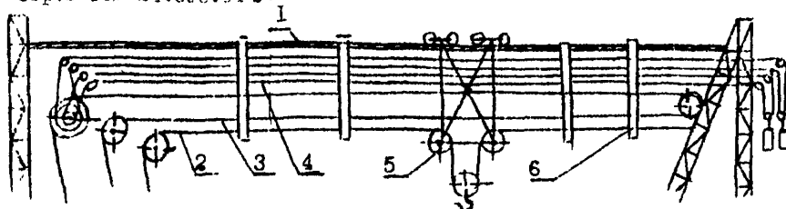
1-несущий канат; 2-подъемный канат; 3-тяговый канат для передвижения грузовой тележки; 4-тяговый канат для передвижения поддержки; 5-грузовая тележка; 6-поддержка приводная.
