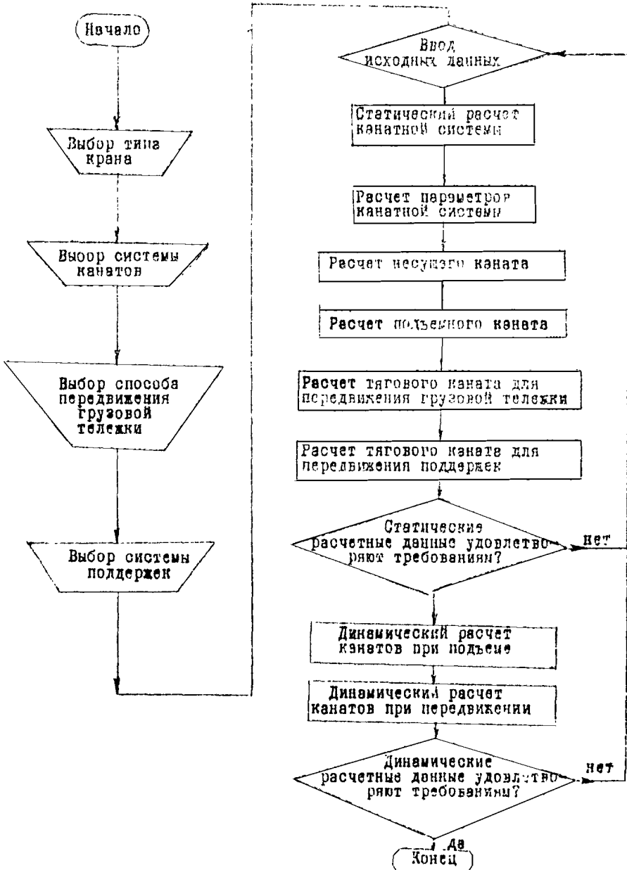
Блок-схема для расчета канатов на ЭЦВМ черт.41
