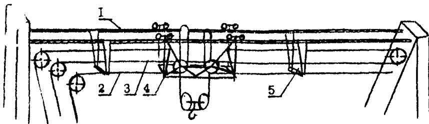
1-несущий канат; 2-подъемный канат; 3-тяговый канат для передвижения грузовой тележки; 4-грузовая тележка; 5-поддержка подвижная открытая
